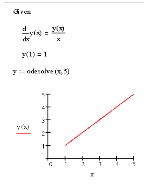
Рис. 2. Використання блоку Given-odesolve
