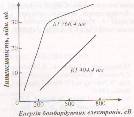
Рис.3. Залежність інтенсивності спектральних ліній КІ 404,4 нм і КІ 766,4 нм від енергії бомбардуючих електронів ( j=1 \text{ мА/см}^2 ).
