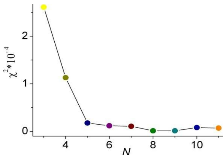
Рисунок 1 – \chi^2 для хвильової функції дейтрона u(r)
