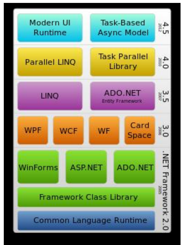
Рис. 6. Стек технологій .NET Framework
