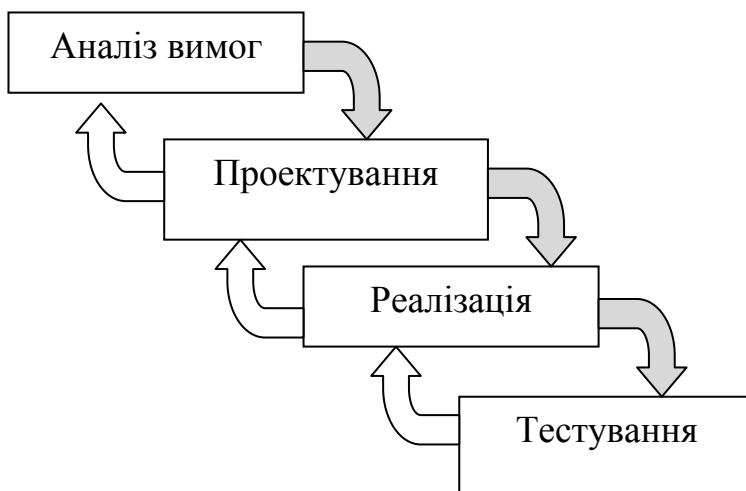
Рис. 2. Водоспадна модель із зворотнім зв'язком
