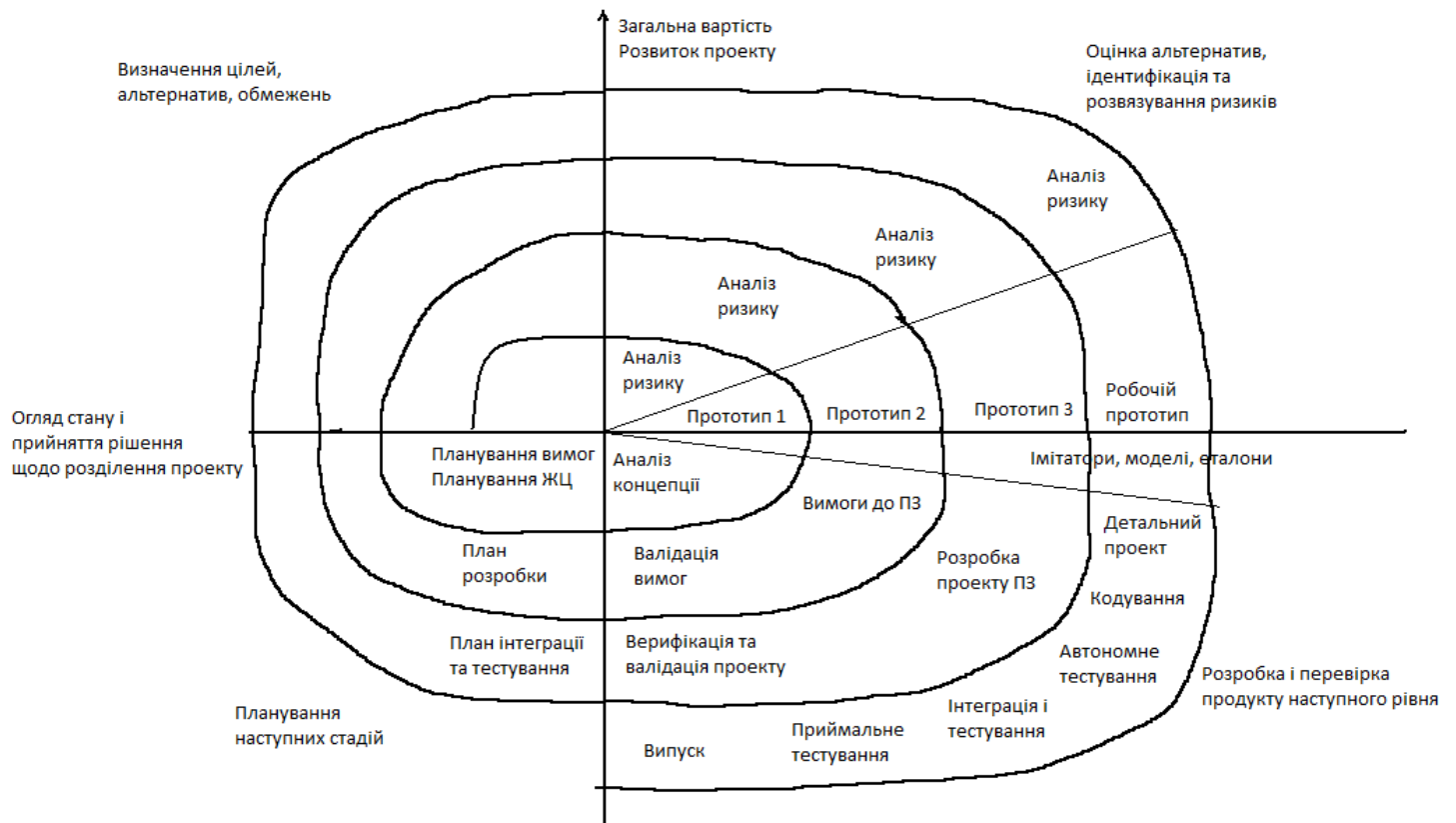
Рис. 4. Спіральна модель
