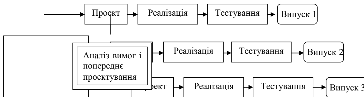
Рис. 3. Ітераційна модель з перекриттям ітерацій
