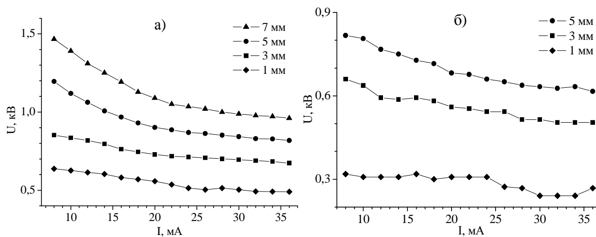
Рис. 5. Вольт-амперні характеристики для розряду на основі дистильованої води: а) водяний катод, б) водяний анод
