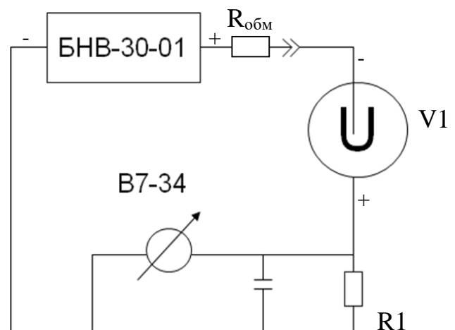
Рис. 2. Узагальнена схема включення датчика: БНВ-30-01 – джерело високої напруги; R обм – обмежуючий резистор; B7-34 – цифровий вольтметр-електрометр; V1 – пропорційний лічильник СИ5007; R1 – вимірювальний резистор 2,0 МОм; C1 – інтегруючий конденсатор
