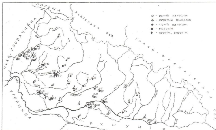
Рис. 1.1. Найдавніші стоянки первісної людини на території Закарпаття. Пам'ятки раннього палеоліту: 1- Мала Бігань, 2–5 – Малий Раковець; 6-12 – Королево; 13–16 Рокосово [139].
