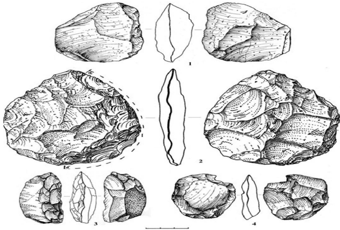
Рис. 1.4. Середньо-палеолітичні знаряддя первісної людини з двобічною обробкою, що знайдені на території с. Рокосово: 1,3 – пункт II; 2 – пункт VI; 4 – пункт III [16, 17].
