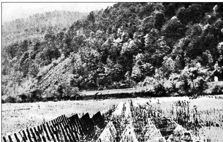
Протитанкові загородження у долині між горами на лінії «Арпада». 1944 р.
