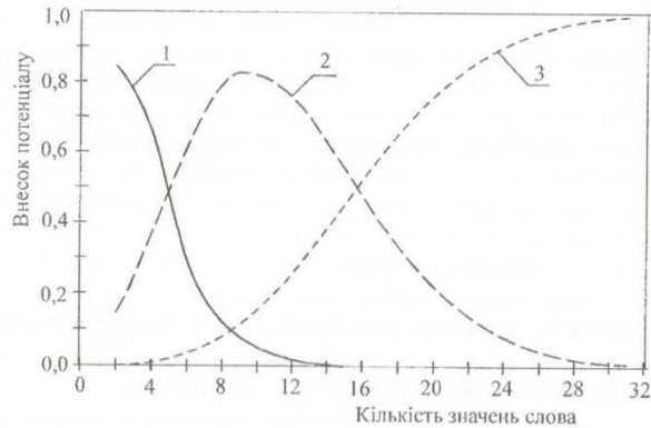
Рис. 2. Графіки внеску окремих експонент у загальну криву, програма ORIGIN 7: 1 – внесок першої експоненти; 2 – внесок другої експоненти; 3 – внесок третьої експоненти
