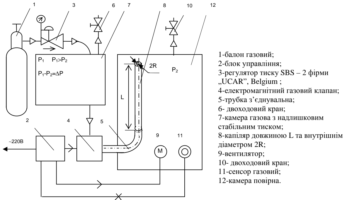
Рис.2. Схема комбінована газова.
