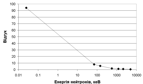
Рис. 2. Залежність відгуку ТЛ елемента на основі ^6\text{LiF} від енергії нейтронів. За одиницю взято відгук на нейтронне опромінення ^{252}\text{Cf} .
