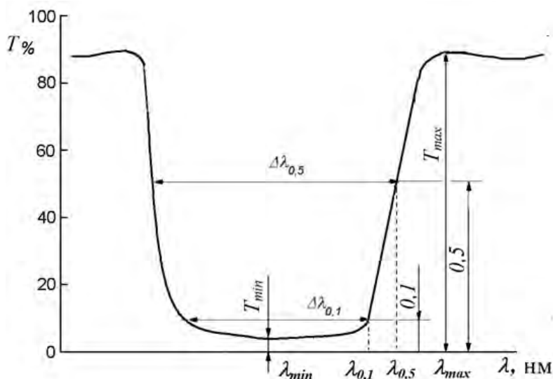
Рисунок 1. Основні характеристики відрізаючих оптичних фільтрів
