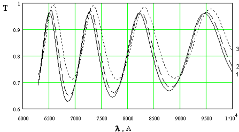
Рис.2. Криві пропускання при різних товщинах d окисного шару: 1 – d=100 А, 2 – d=200 А, 3 – d=300 А.
