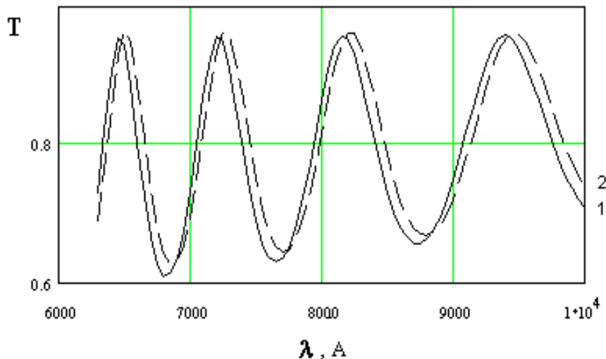
Рис. 1. 1 – підкладинка, n_0=1.51 ; шар As_2S_3 має дисперсію: при \lambda=6300 А, n=2.6 , при \lambda=10000 А, n=2.3 , геометрична товщина шару d=10000 А; 2 – наявний шар-окислу: n=1.8 , d=200 А.
