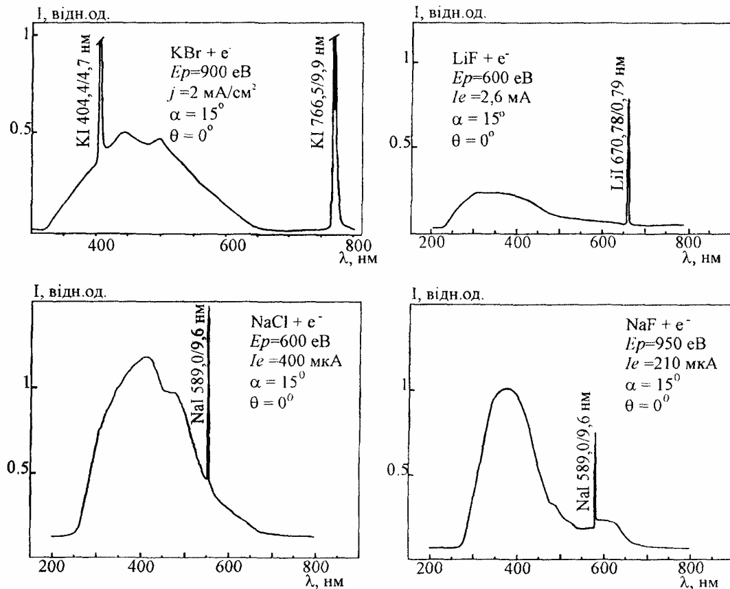
Рис. 1. Спектрограми свічення деяких ЛГК при бомбардуванні електронами.
