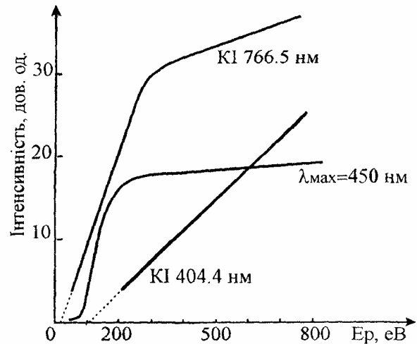
Рис. 3. Залежності інтенсивності ліній KI 766,5 нм і KI 404,4 нм від енергії первинних електронів для кристала KBr.
