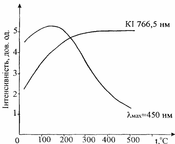
Рис. 4. Залежність інтенсивності дублету ліній KI 766,5/6,9 нм та смуги випромінювання з максимумом при 450 нм від температури мішені.
