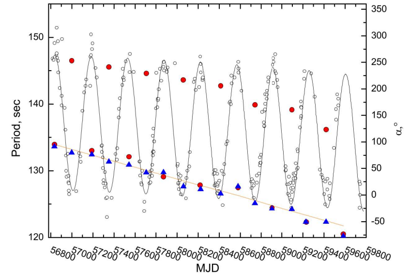
Рис. 2.5. Залежність зміни періоду власного обертання супутника “MIDAS-7” від положення Сонця, Місяця і висхідного вузла орбіти супутника, на інтервалі з 2014 по 2022 р. Суцільна лінія - функція 2.1, пунктир - зміна прямого сходження вузла орбіти ШСЗ “MIDAS-7”, біле коло - значення власного обертання ШСЗ “MIDAS-7”, червоне коло - положення Сонця, синій трикутник - положення Місяця
