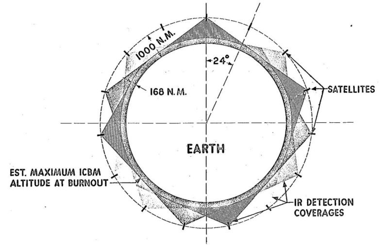
Рис. 2.1. Розташування та покриття супутників серії “MIDAS” 1957 рік [17]
