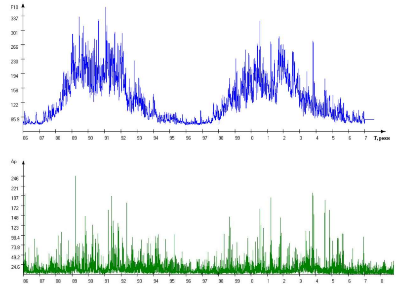
Рис. 4.4. Зверху: зміни потоку радіовипромінювання Сонця на \lambda = 10.7\text{см} (F10.7) в період з 1986 по 2008 рр. Знизу: зміни геомагнітного індексу (Ap) в період з 1986 по 2008 рр.
