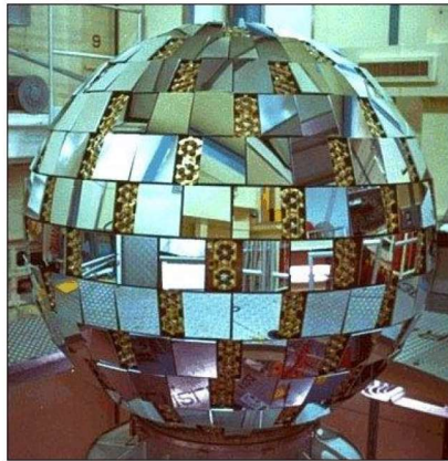
Рис. 4.1. Геодезичний супутник “Ajisai”, та Схематичний розподіл його панелей LLR
