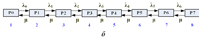
Рис. 3. Моделі функціонування п'ятирангової мережі: а – поярусна, б – «загибелі та розмноження»
