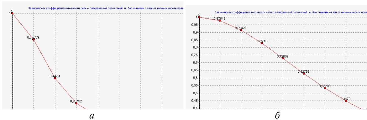
Рис. 4. Графік залежності коефіцієнта готовності з п'ятьма ВК і топологією «кільце» від інтенсивності збоїв ( \lambda_3 = 0,05 для критерію зв'язності \geq 1 ): а) \mu_e = 0,4 ; б) \mu_e = 1,4 .
