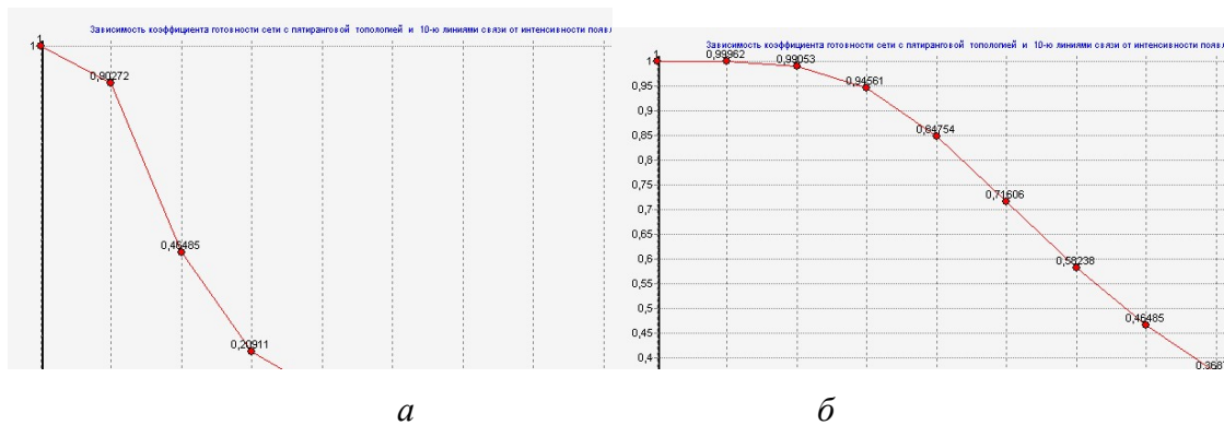
Рис. 5. Графік залежності коефіцієнта готовності з п'ятьма ВК топології «повна сітка» ( \lambda_3 = 0,05 для \geq 1 ): а) \mu_e = 0,4 ; б) \mu_e = 1,4 .
