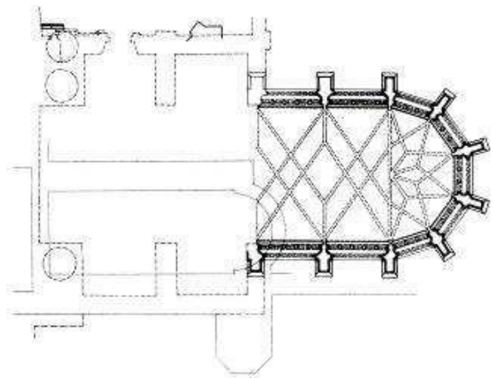
24. Praha. Hrad. Kaple Věšch svatých. Pohled od jihu, půdorys – částečná rekonstrukce a pohled do nitra - rekonstrukce. Před 1380.
