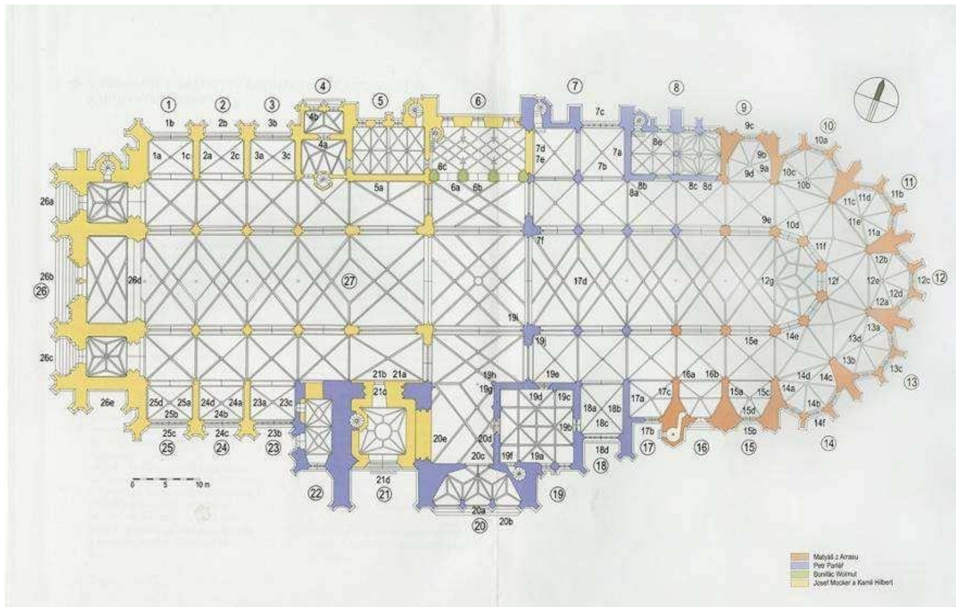
12. Praha. Katedrála sv. Víta. Půdorys s vyznačením stavebních etap (položení základního kamene 21. listopadu 1344).
