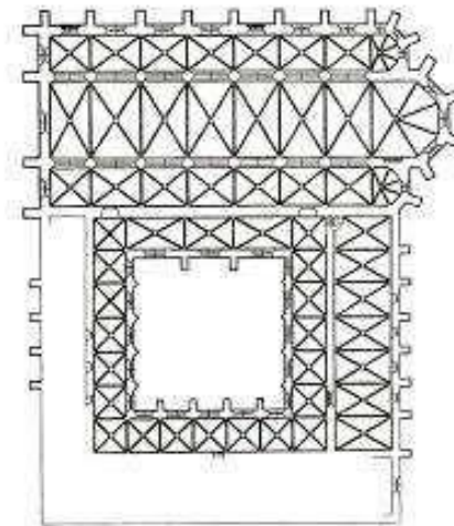
28. Praha. Nové Město. Klášter slovanských benediktinů v Emmauzích. Pohled od východu, interiér kostela a půdorys. (založení kláštera r. 1347, svěcení klášterního kostela r. 1372).
