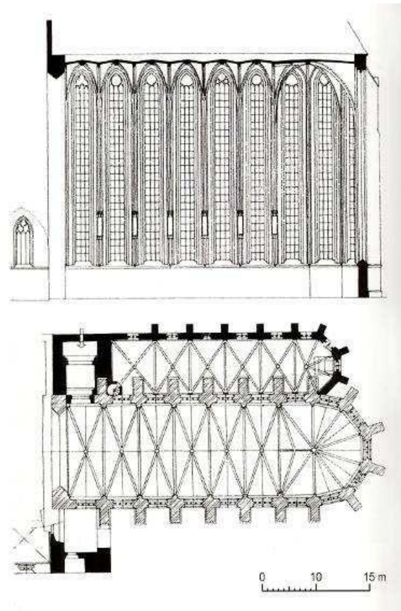
27. Praha. Nové Město. Bývalý klášter karmelitánů. Kostel P. Marie Sněžné. Pohled od jihu, půdorys a podélný řez (založení kláštera r. 1347).
