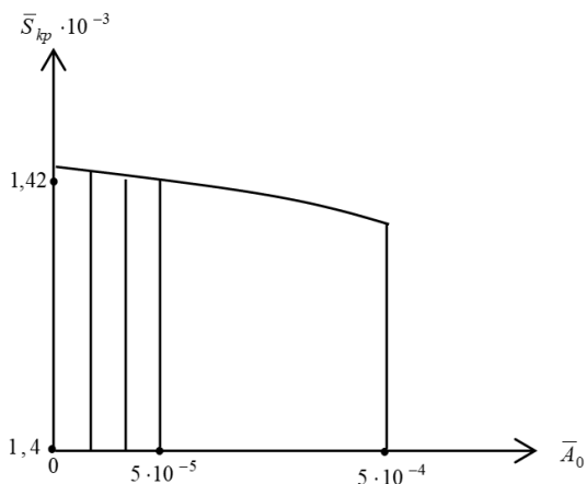
Рис. 5. \bar{S}_{кр} = \bar{S}_{кр}(\bar{A}_0) для круглой пластинки из стали SAM 316 и при \gamma = 0,02 .
