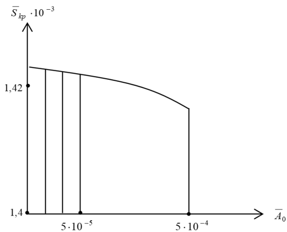
Рис. 3. \bar{S}_{кр} = \bar{S}_{кр}(\bar{A}_0) для круглой пластинки из стали SW 316 и при \gamma = 0,02 .
