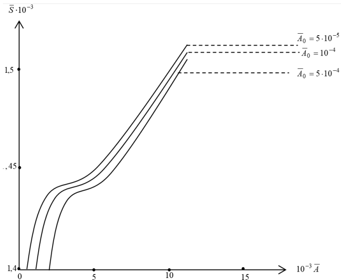
Рис. 4. Зависимость \bar{S} = \bar{S}(\bar{A}) в различных значениях начального пригиба \bar{A}_0 (SAM 316).
