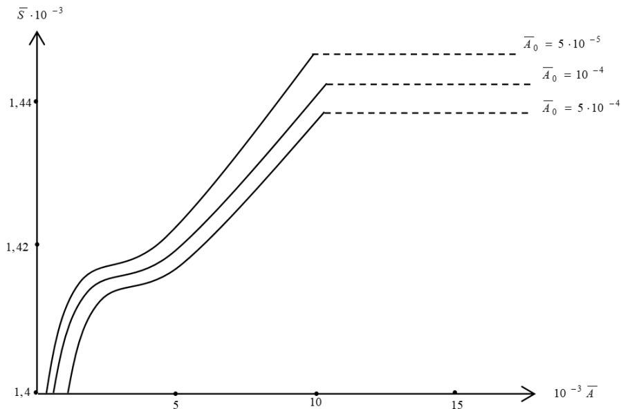
Рис. 2. Зависимость \bar{S} = \bar{S}(\bar{A}) в различных значениях начального пригиба \bar{A}_0 (SW 316).
