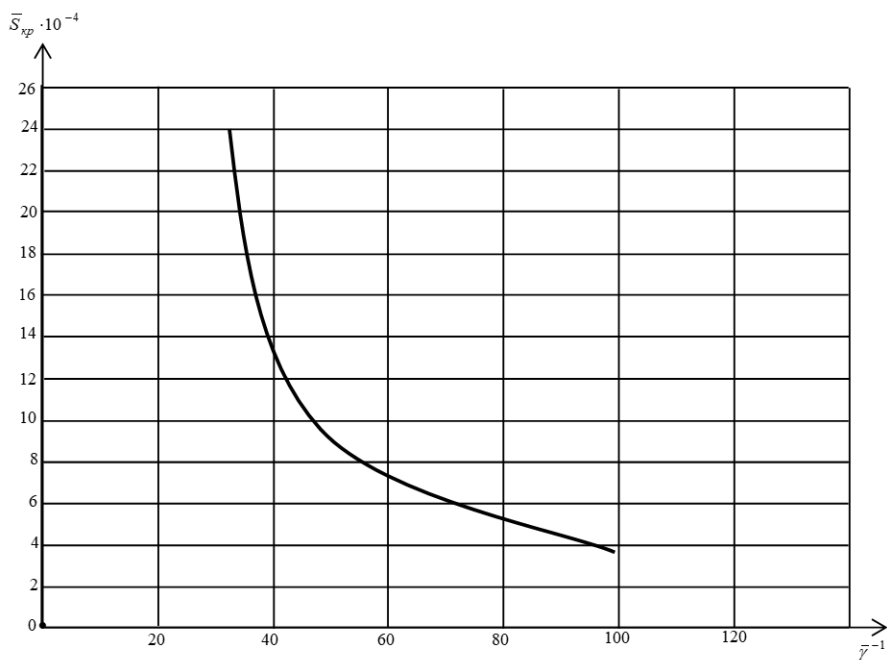
Рис. 1. Зависимость критического объемного распухания от относительной толщины для пластинки при \bar{A}_0 = 10^{-4} .
