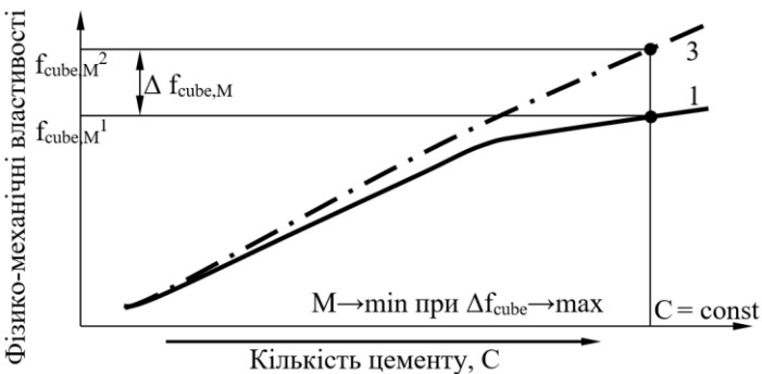
Рис.1 – Вплив витрат цементу на зміну матеріалоемкості:
