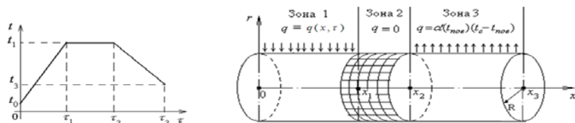
Рис. 1. Графік термообробки та трьохзонна модель місцевого нагріву
