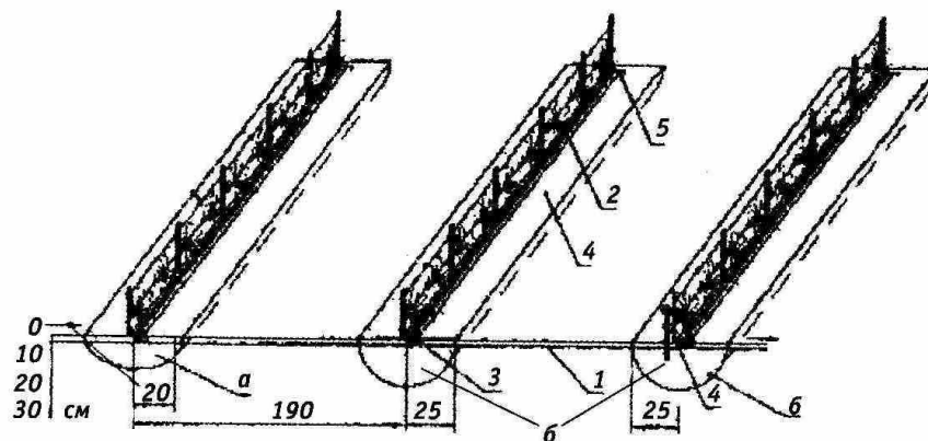
Рис. 5. Формування зони зволювання на суглинистих ґрунтах при крапельному зрошенні огірка на шпалері із широкорядним (190×25 см) висівом (посадкою). Зволювання площі – 31%: 1 – дільничний трубопровід; 2 – поливний плівковий трубопровід; 3 – з’єднувачі; 4 – тензіометр; 5 – заглушка поливного трубопроводу; 6 – смуга зволювання ґрунту; а – в перший період вегетації; б – у другий період вегетації
