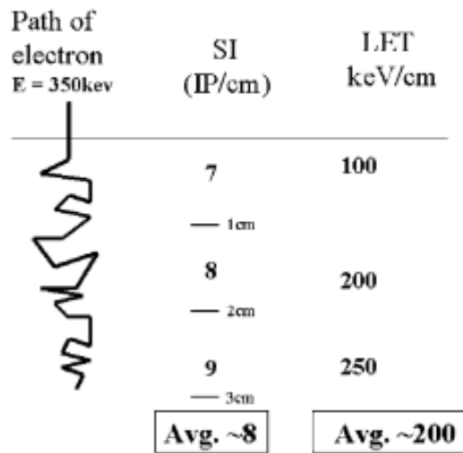
Рисунок 4. Схематичне зображення траєкторії високоенергетичних електронів (бета-часток) у речовині.
