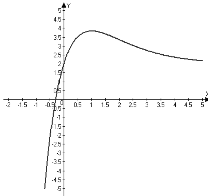
Рис. 1. Графік функції y = 5xe^{-x} + 2 .
