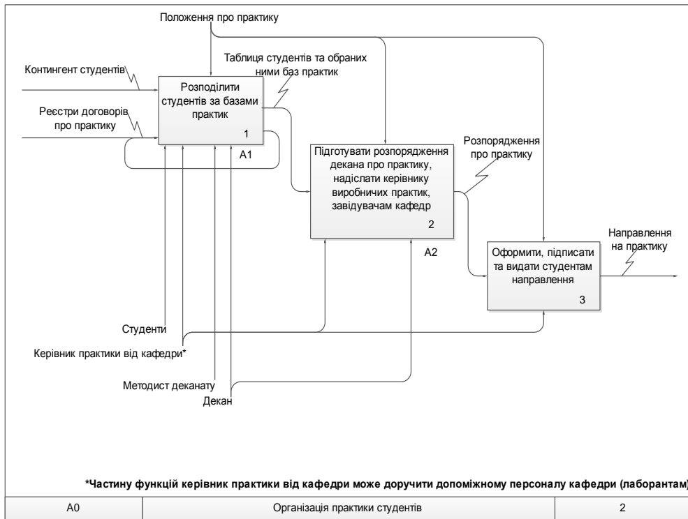
Рис. 8. Організація практики студентів – перший рівень декомпозиції, ТО-VE*
