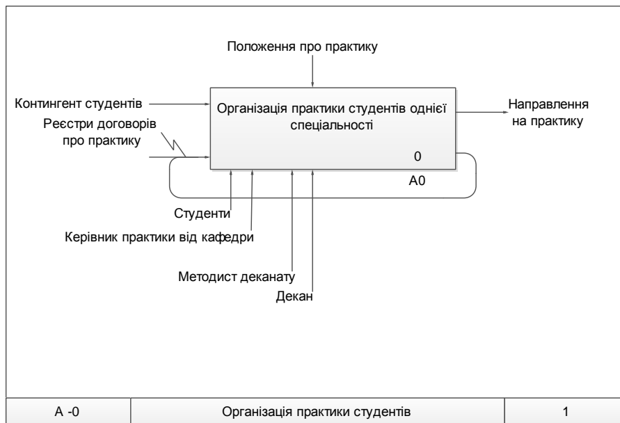
Рис. 9. Організація практики студентів – контекстна діаграма, ТО-VE*
