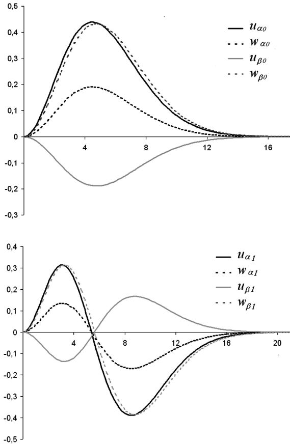
Рис. 1. Радіальні хвильові функції основного ( n=0 ) та першого збудженого ( n=1 ) станів. В \alpha -стані переважає синглетна компонента хвильової функції, в \beta -стані – триплетна.
