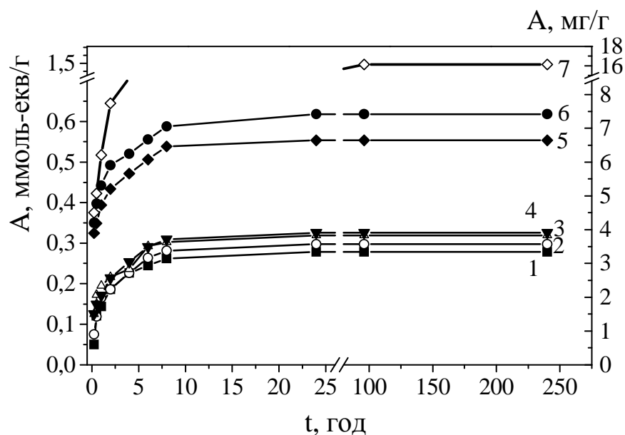
Рис. 1. Залежність величини сорбції (А) йонів магнію від часу контактування на досліджених цеолітах: 1 – природний морденіт; 2 – природний кліноптилоліт; 3 – калієва форма морденіту; 4 – калієва форма кліноптилоліту; 5 – натрієва форма морденіту; 6 – натрієва форма кліноптилоліту; 7 – синтетичний цеоліт NaX.
