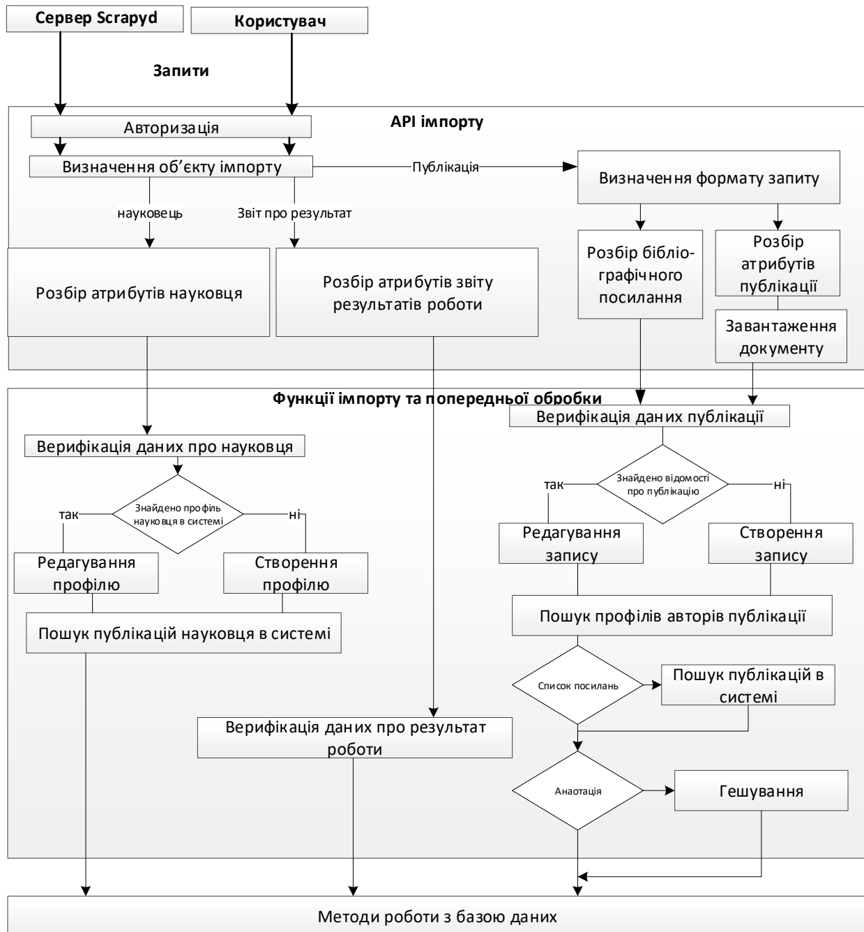
Рисунок 6 – Алгоритму функціонування модулю імпорту
