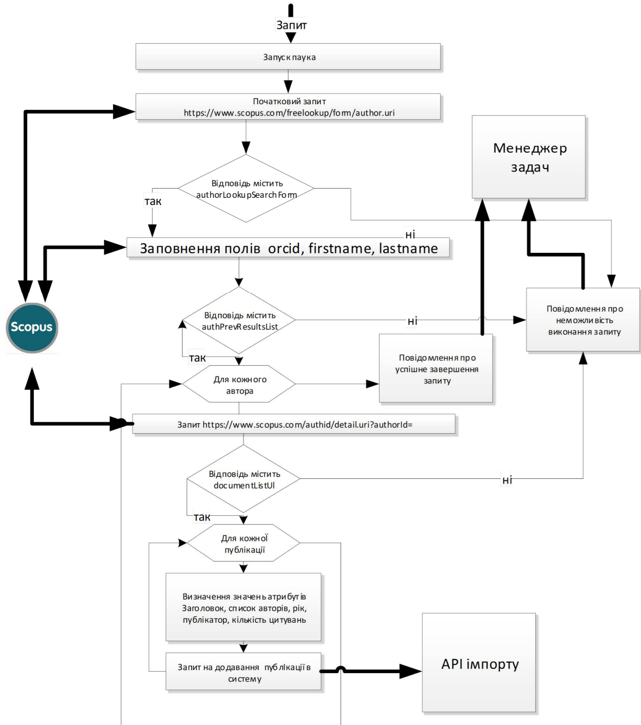
Рисунок 5 – Алгоритм скрапінгу інформації про публікації науковця на прикладі наукометричній базі SCOPUS
