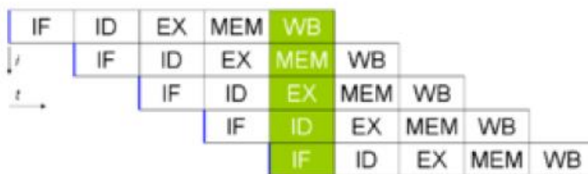
Рис. 2.5. Стандартний п'ятикроковий конвеєр в машині RISC.
