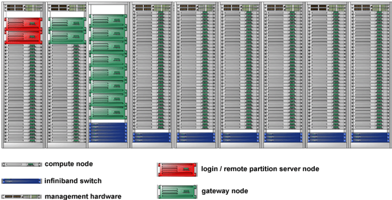
Рис. 1.6. Схема будови кластера LLNL
