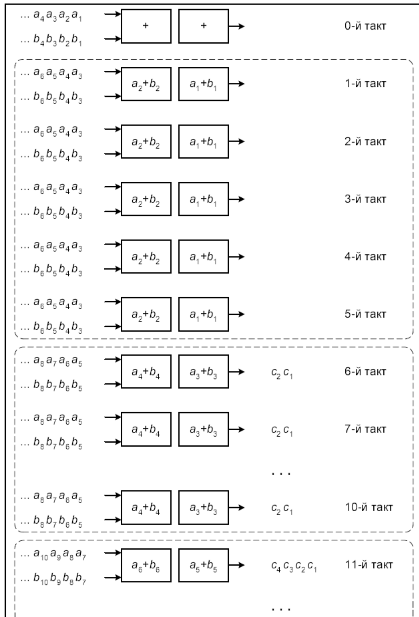
Рис. 2.4. Паралельне додавання векторів на двох однакових пристроях
