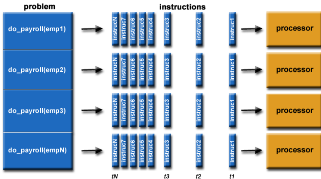
Рис. 1.4. Схема паралельного обчислення зарплати
