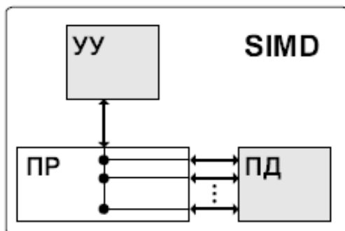
Рис. 2.9. Клас SIMD класифікації Флінна
