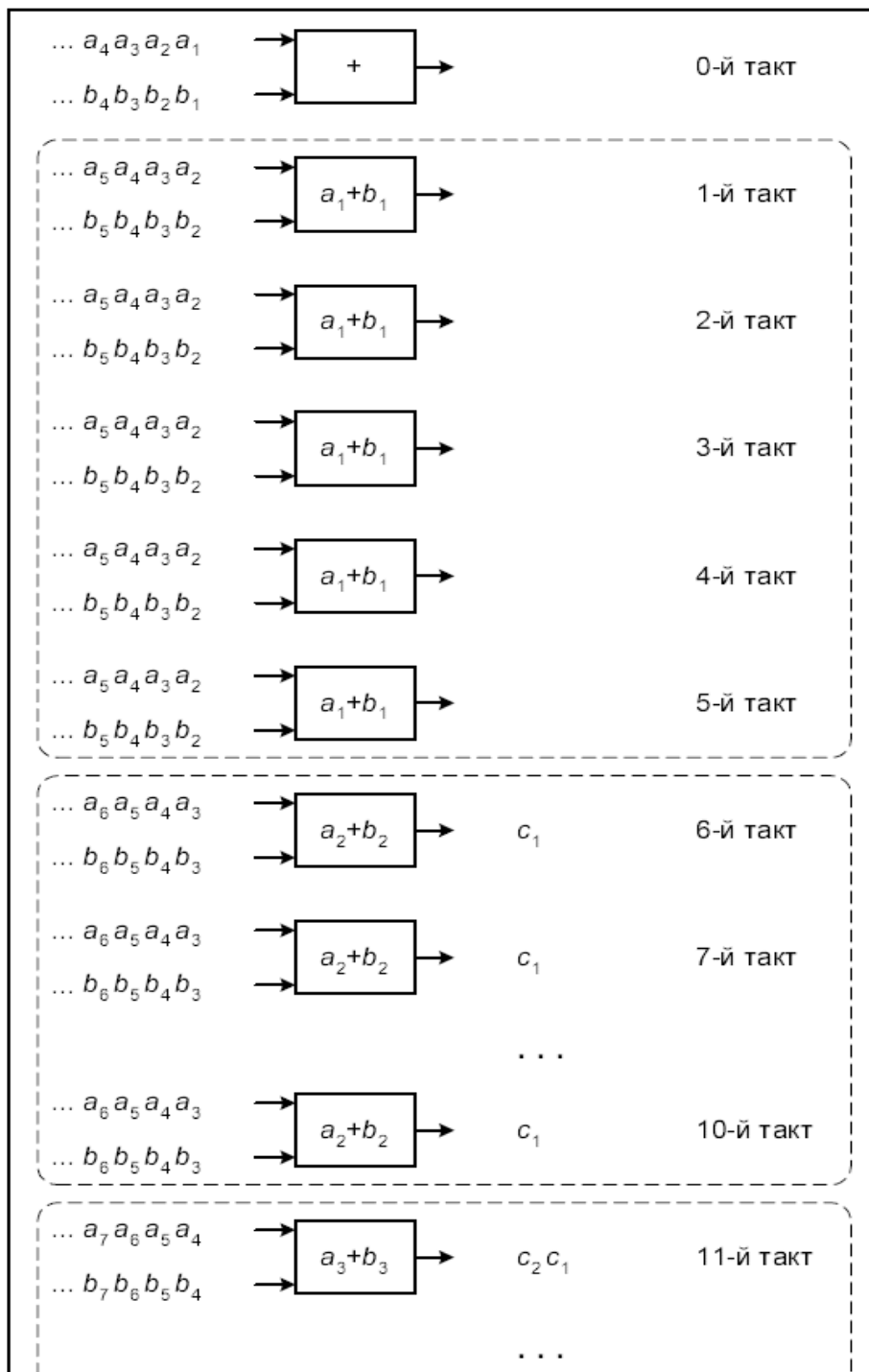
Рис. 2.3. Додавання векторів на послідовному пристрої з 5-тактовою операцією додавання
