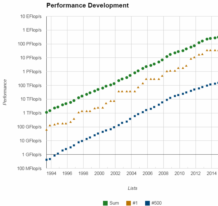
Рис. 1.7. Зростання продуктивності суперкомп’ютерів (за даними Top500.org ).
