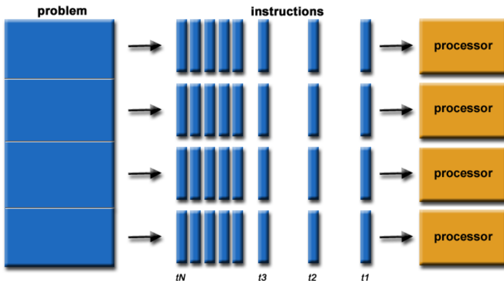
Рис. 1.3. Схема паралельних обчислень
