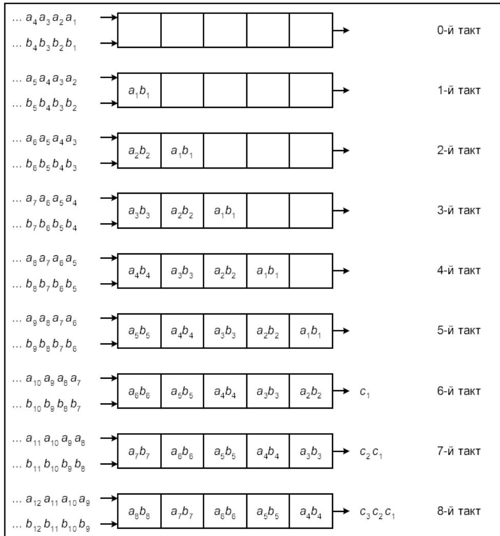
Рис. 2.6. Знаходження суми c = a + b за допомогою 5-стадійного конвеєрного пристрою
