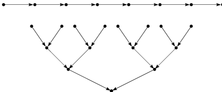
Рис. 3.1. Послідовний граф та граф алгоритму "здвоєння"
