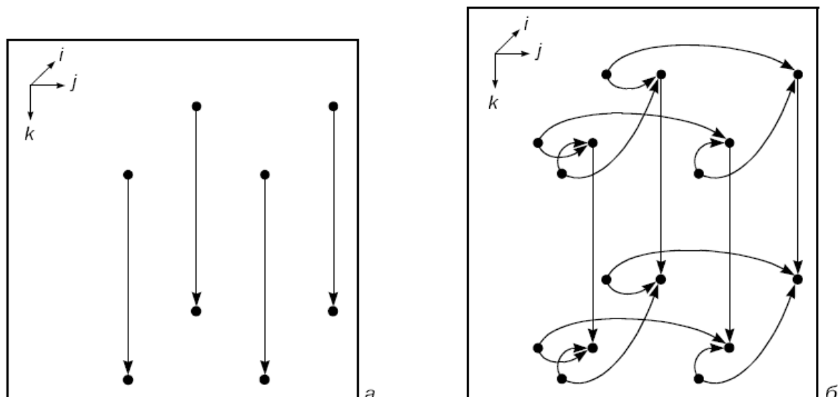
Рис. 3.2. Граф алгоритму множення матриць
