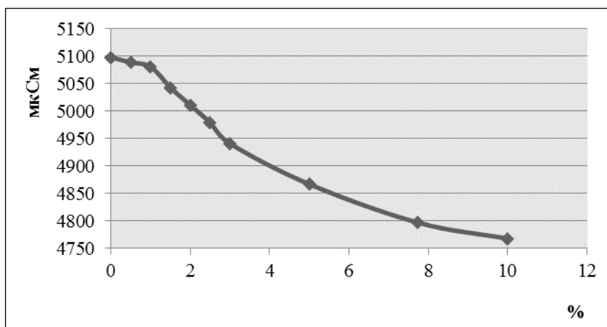
Рис. 2. Зміна електропровідності молока при його фальсифікації водою
