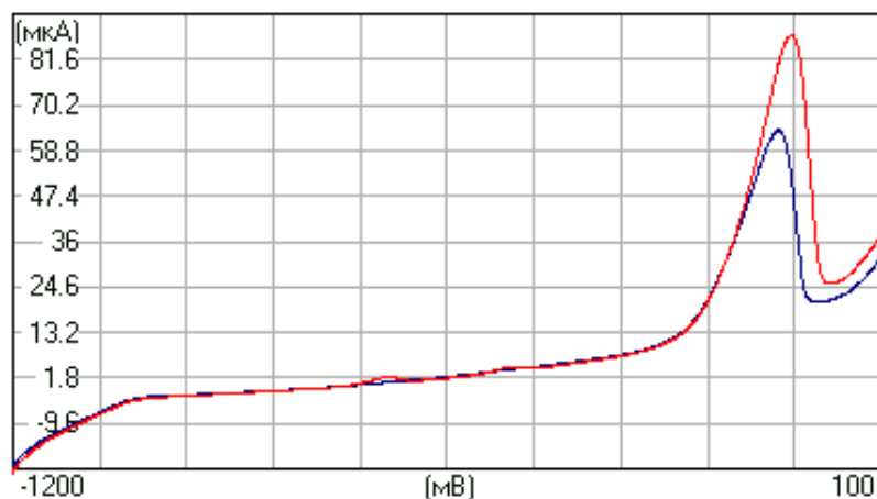
Рис. 1. Вольтамперограма токсичних елементів у зразках хліба пшеничного
