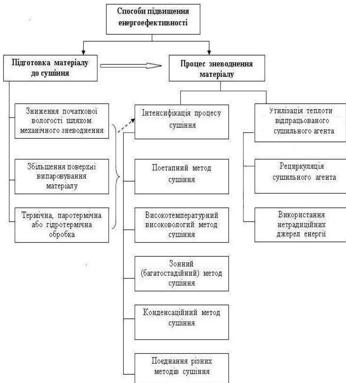
Рис. 2. Напрями підвищення ефективності конвективного сушіння
