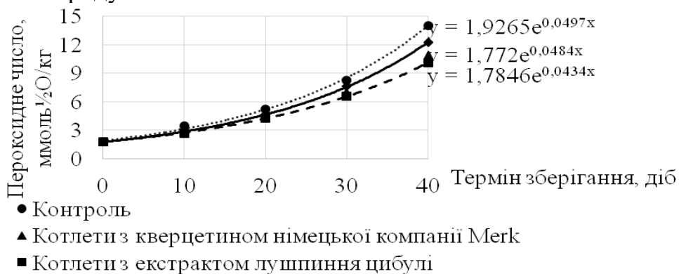
Рис. 5. Динаміка змін пероксидного числа напівфабрикатів, ммоль ^{1/2} О/кг ( t_{\text{зберіг.}} -12\text{ }^{\circ}\text{C} , p \leq 0,05 )
