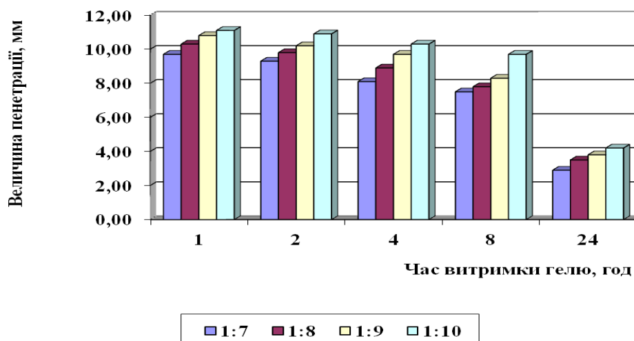
Рис. 2. Залежність величини penetрації від ступеня гідратації і часу витримки гелю
