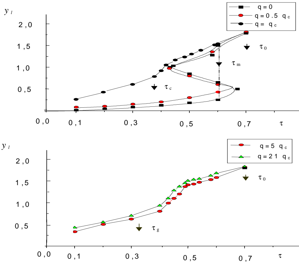
Рис. 2. Температурна залежність приведених середньоквадратичних зміщень атомів вздовж зв'язку y_l при різних швидкостях охолодження q .
