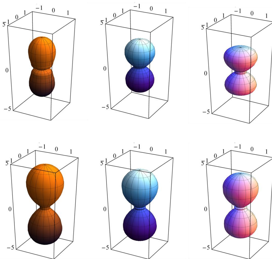
Рис. 3. Угловые распределения электрона e_2 в ПДИ для различных конечных состояний Ne^{2+}(2p^4\ ^1S, ^1D, ^3P) при энергиях фотонов 27.8 эВ (верхний ряд) и 51.15 эВ (нижний ряд), соответствующих прямой двухфотонной и двухфотонной надпороговой ионизации Ne^+(2p^5\ ^2P_{3/2}) , соответственно. Вектор линейной поляризации направлен вертикально. Нормировочный множитель один и тот же для всех угловых распределений.
