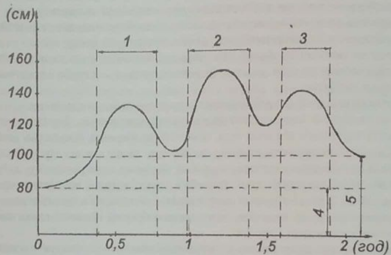
Рис. 9. Схематичне зображення біоенергетичних процесів
