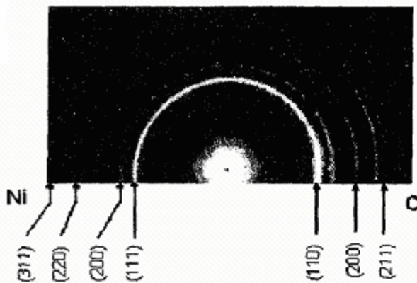
Рис.4. Електроннограма для невідпаленої плівки Ni(15nm)/Cr(25nm)/П.
