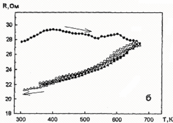
Рис.5. Залежність R(T) для трьох циклів "нагрівання↔охолодження" для плівок Ni(15нм)/Cr(25нм)/П (а), Cr(90нм)/Co(40нм)/П (б): ○, ● – I цикл; □, ■ – II цикл; ▲, △ – III цикл.
