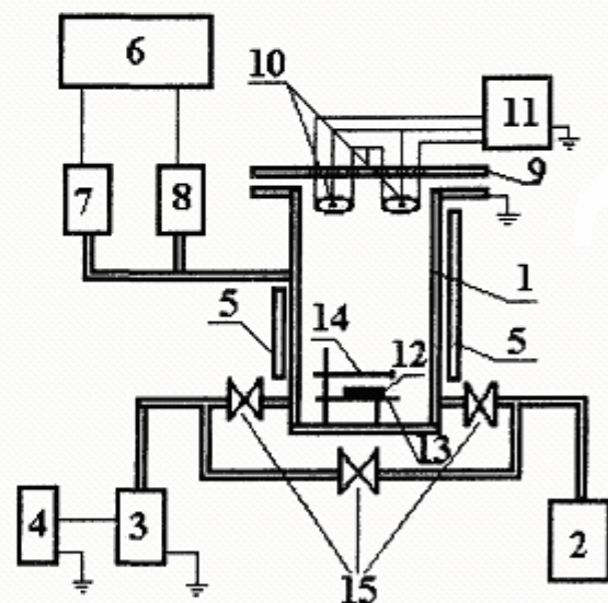
Рис. 1. Блок-схема високовакуумної установки:
