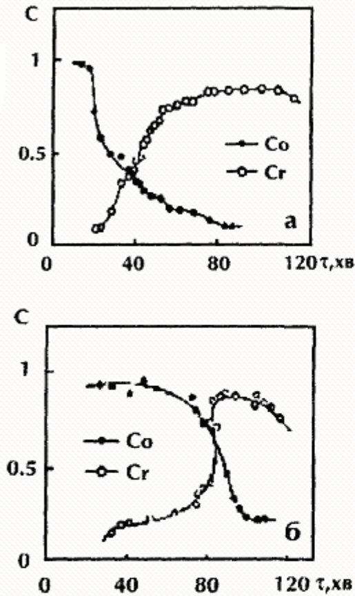
Рис.3. Дифузійні профілі для невідпаленої (а) та відпаленої (б) плівкової системи Co(4000nm)/Cr(2000nm)/П.
