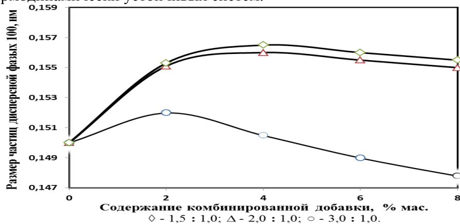
Рис. 2. Размер частиц дисперсной фазы битумов, модифицированных комбинированными добавками (Р+ГПС)
