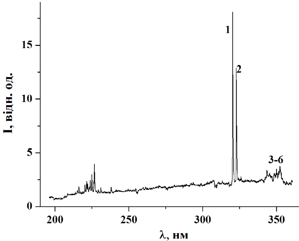
Рис. 4: Спектр випромінювання перенапруженого наносекундного розряду між мідними електродами в аргоні при p(\text{Ar}) = 50 кПа ( d=2 мм).
