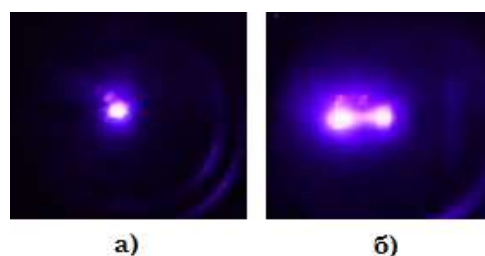
Рис. 1: Світлини перенапруженого наносекундного розряду між мідним і цинковим електродами при p(\text{Ar}) = 50 кПа ( d=2 мм) а), і p(\text{Ar}) = 100 кПа ( d=2 мм) б).
