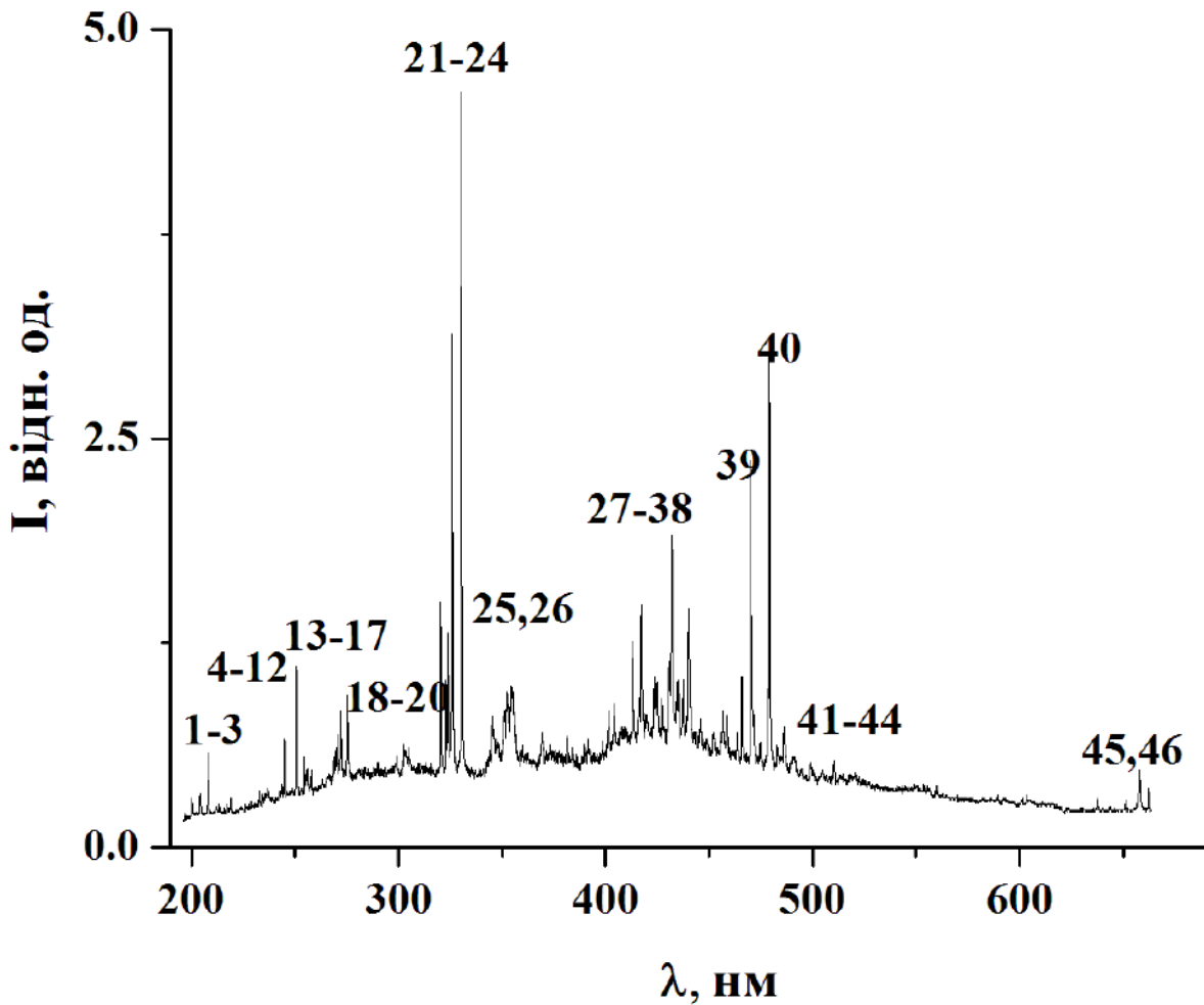
Рис. 5: . Спектр випромінювання плазми перенапруженого наносекундного розряду між електродом з міді і електродом з цинку при p(\text{Ar}) = 50 кПа ( d=2 мм).
