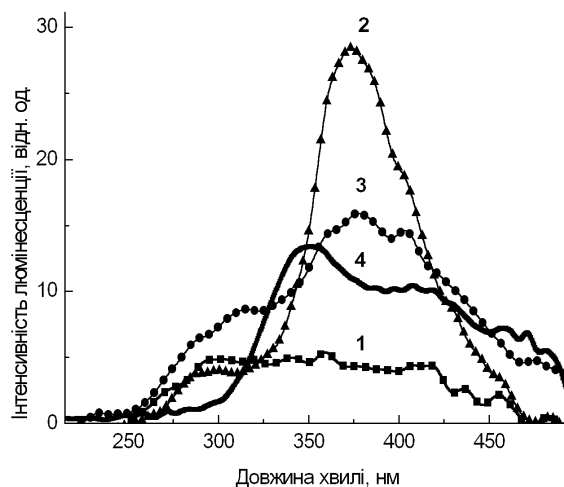
Рис. 1. Спектр рентгенолюмінесценції монокристала \text{Li}_2\text{B}_4\text{O}_7 (1), монокристалів \text{Li}_2\text{B}_4\text{O}_7:\text{Cu} (2, 3) та спектр катодолумінесценції монокристалів \text{Li}_2\text{B}_4\text{O}_7:\text{Cu} (4).
