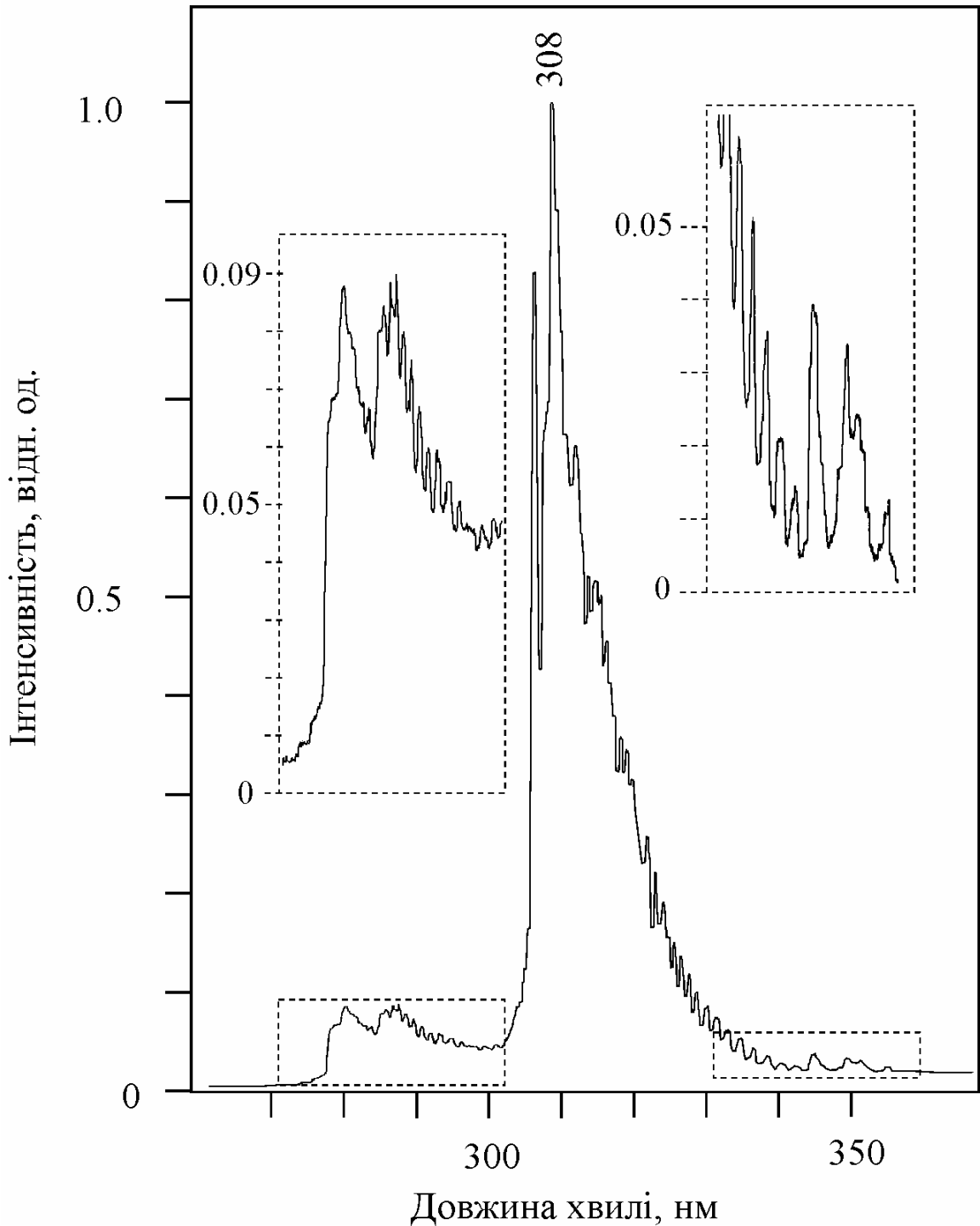
Рис.2. Спектр випромінювання смуг електронного переходу X^2\Pi - A^2\Sigma^+ молекули OH з катодної плями.
