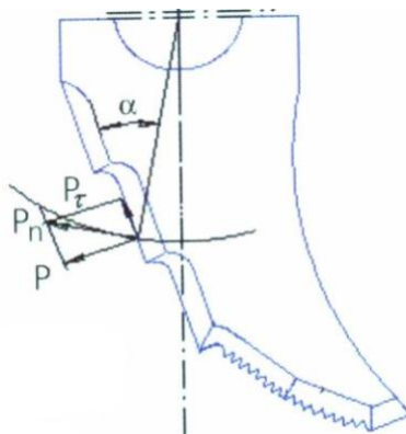
Рис. 5. Кутерний ніж з лінією леза у вигляді зубчатої лінії
