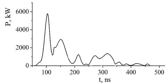
Рис. 1. Імпульсна потужність перенапруженого наносекундного розряду між двома електродами, виготовленими з халькопіриту при: p(\text{Ar}) = 101 кПа
