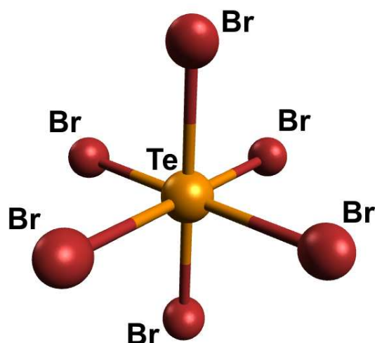
Рис. 1. Загальний вигляд структури [\text{TeBr}_6]^{2-} аніона.
