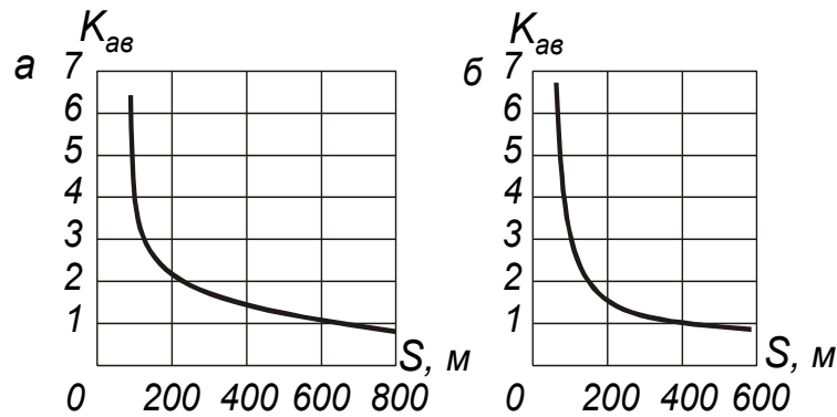
Рис. 1. Залежність коефіцієнту аварійності від відстані видимості:
