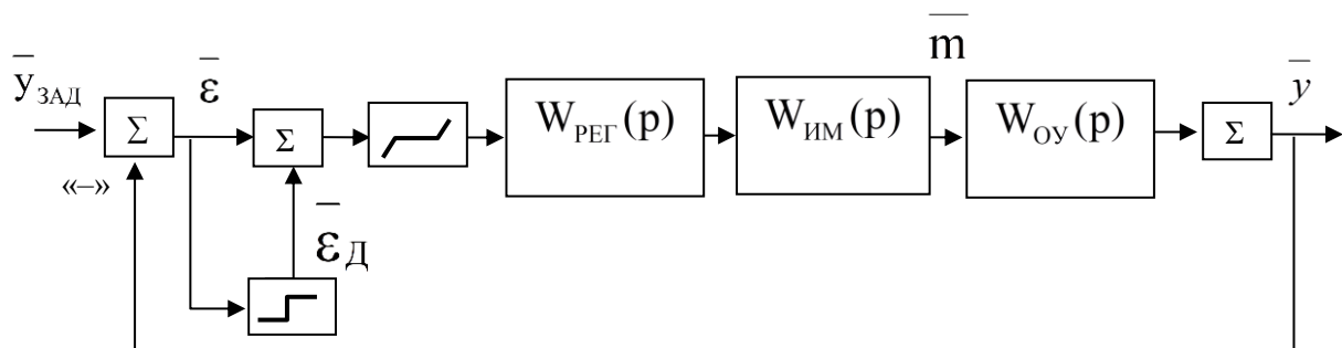
Рис. 1 Структурно-динамічна схема САР
