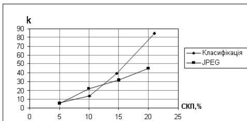
Рис. 2. Залежність коефіцієнта стиску k від СКП при кодуванні зображення мазку крові (*.bmr) методом автоматичної класифікації при m=4 и k=80 і стандартним методом JPEG.
