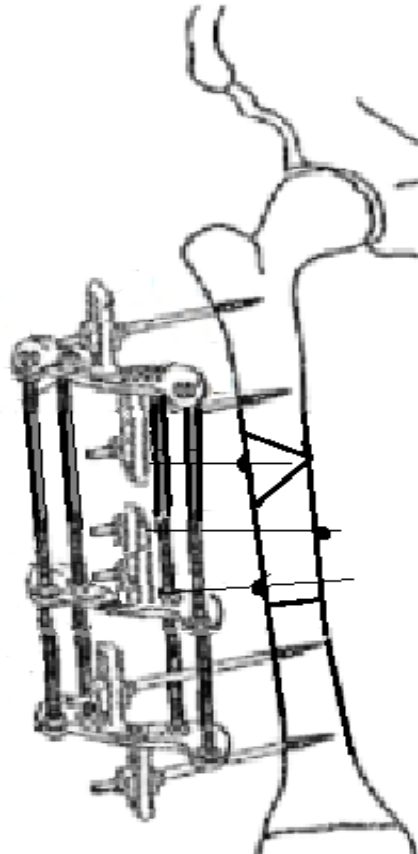
Рис. 1. Общая схема проведения спиц с упорными площадками
