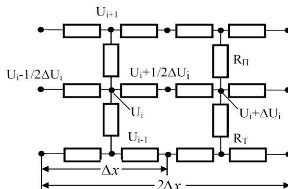
Рис. 1. Електрична схема відрізків i – того та i + 1 тросів
