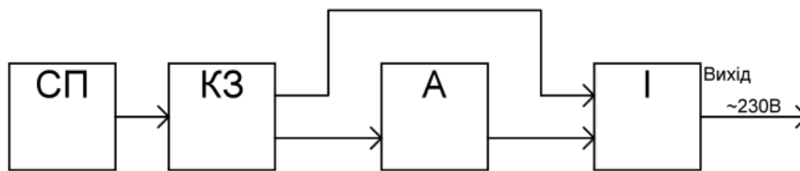
Рис. 1. Структурна схема класичної автономної сонячної електростанції. Де СП – сонячна панель, КЗ – контролер заряду, А – акумулятор, І – інвертор.
