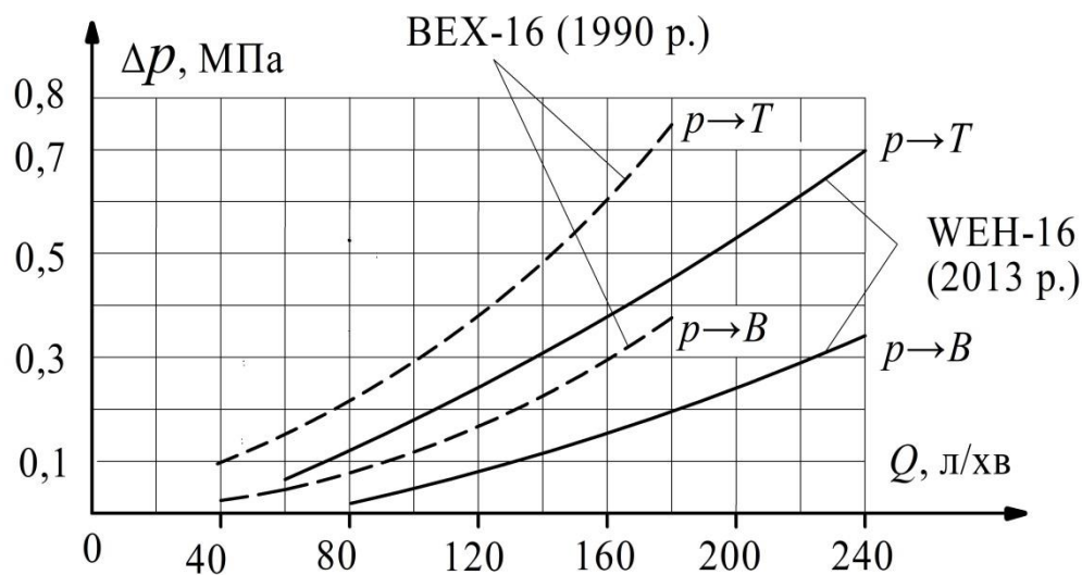
Рис. 1. Втрати тиску від витрати в гідророзподільниках різних років виробництва (при однаковій в'язкості РР в 41 мм 2 /с)
