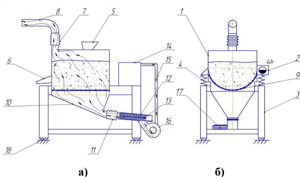
Рис. 1. Конструктивна схема віброозонуючого комплексу періодичної дії для сушіння зернової сировини а – вигляд спереду; б – вигляд збоку;
