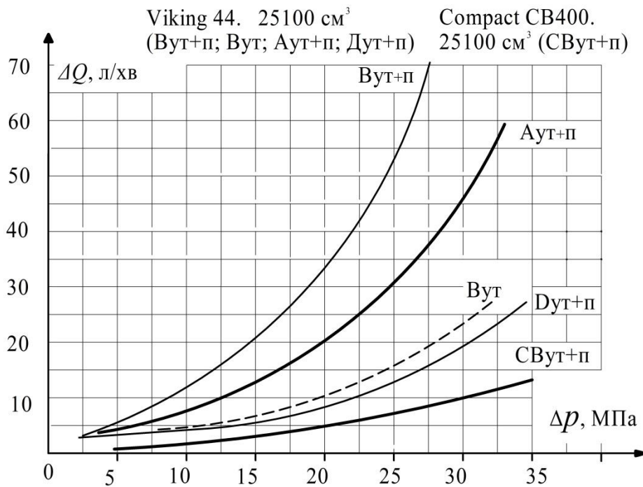
Рис. 2. Зміна об'ємних втрат у радіальнопоршневих гідромоторах VIKING44 та COMPACT-CB400 з однаковим робочим об'ємом 25100 см 3 залежно від тиску і при постійній в'язкості РР у 40 сСт (мм 2 /с)
