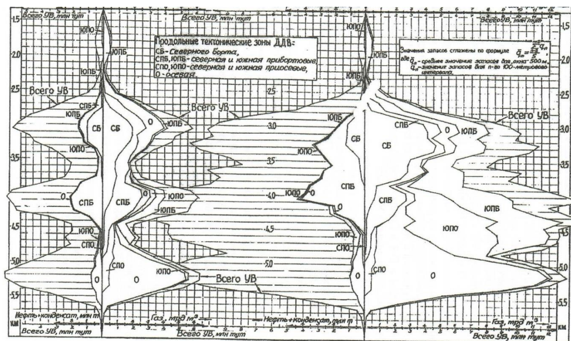
Рис. 3. Распределение начальных извлекаемых запасов нефти, газового конденсата и газа по величинам месторождений, фазовому составу, продольным тектоническим зонам и гипсометрическим уровням залегания нижнекаменноугольных отложений в комбинированных ловушках на моноклиналях [6].
