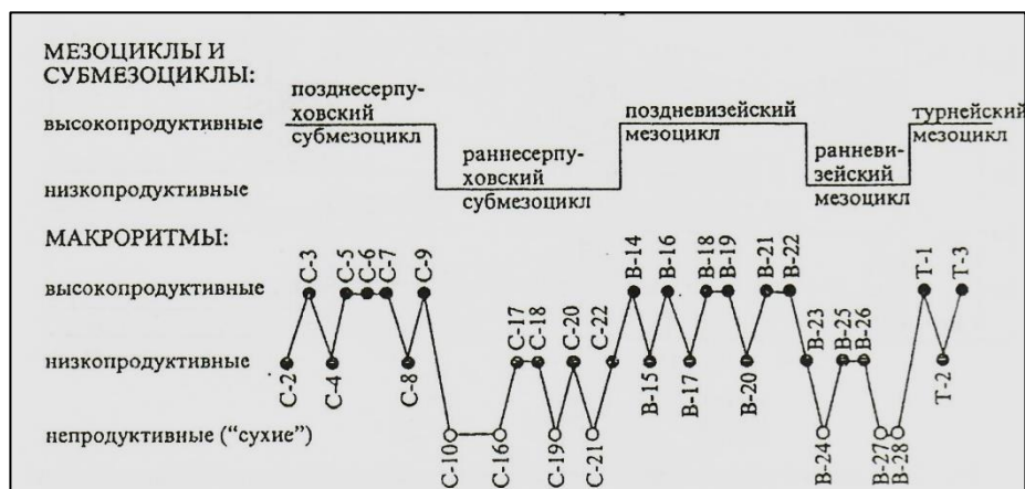
Рис. 2. Схема цикличности нефтегазонакопления раннекаменноугольных мезоциклов и макроритмов в Днепроовско-Донецкой впадине [6].
