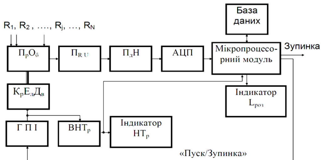
Рис. 2. Структурна схема системи контролю розриву тросів
