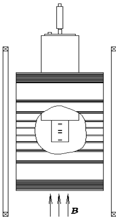
Рис. 3. Балансування надпровідної антени по вертикальній складовій (Z) з встановленим соленоїдом
