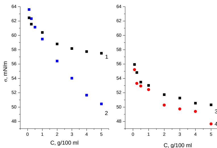
Рис.4. Ізотерми поверхневого натягу полі(2-етилоксазолінів) (1 - M = 600; 3 - M = 2100) та адуктів з пероксидним фрагментом на основі відповідних полі (2-етилоксазолінів)
