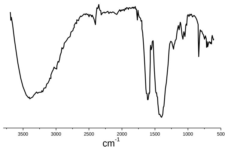
Рис.2. ІЧ-спектр полі(2-етилоксазоліну) з кінцевою пероксидною групою
