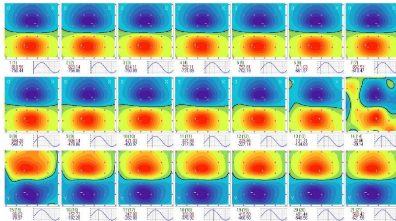
Рис 4. 21 карта магнітного поля тестового зразка збалансованої надпровідної антени
