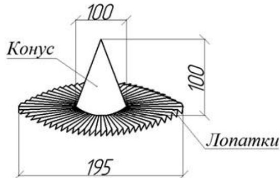
Рис. 1. Принципова схема повітророзподільної насадки.
