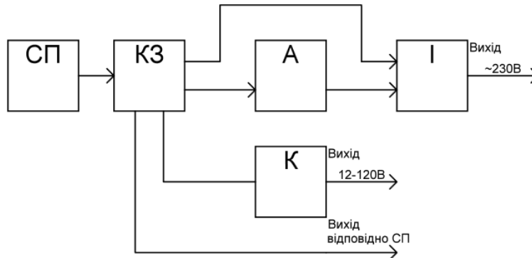
Рис. 2. Структурна схема автономної сонячної електростанції з можливістю відбору електроенергії постійної напруги. Де К – конвертор.
