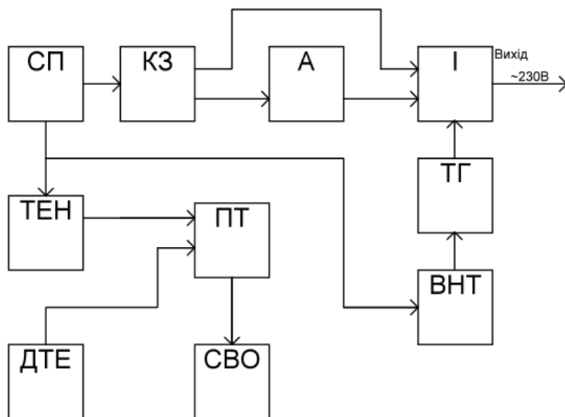
Рис. 4. Структурна схема автономної системи електро- та теплопостачання. Де ТЕН - трубчатий електронагрівач, ПТ - пристрій керування подачею тепла, ДТЕ - регульоване джерело теплової енергії на основі газового, твердопаливного чи рідинного котла, СВО - система водяного обігріву жилих приміщень, ВНТ - вихідний нагрівач тепла з використанням ТЕН, ТГ - термоелектричний генератор.
