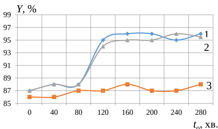
Рис. 2. Схожість отриманої зернової сировини в залежності від концентрації озону 1 – при концентрації озону 10 \text{ мг/м}^3 ; 2 – при концентрації озону 15 \text{ мг/м}^3 ; 3 – при відсутності озону у складі сушильного агенту
