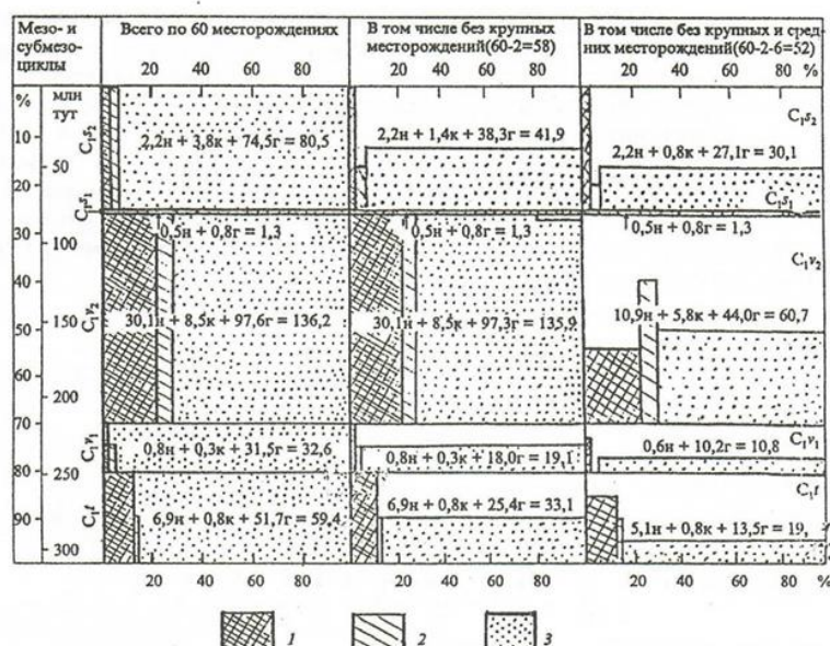
Рис. 1. Диаграмма распределения начальных извлекаемых запасов УВ по мезоциклам нефтегазонакопления в Днепровско-Донецкой впадине [6].
