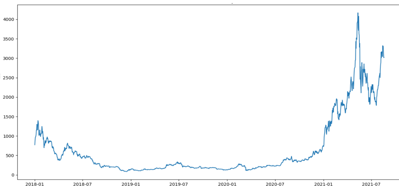
Рис.1. Значения цены закрытия для криптовалют Solana (а) и Ethereum (б) в долларах США (по оси абсцисс располагаются даты, а по оси ординат – цена закрытия).
