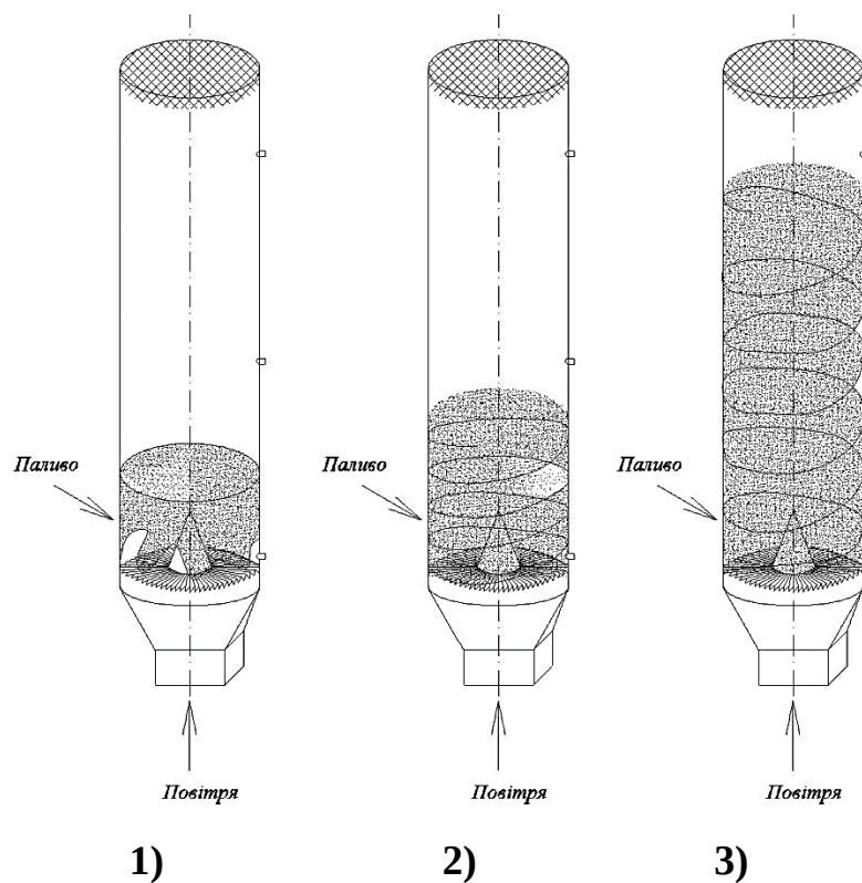
Рис. 2 Характер розповсюдження паливно-повітряної суміші за різної витрати повітря.
