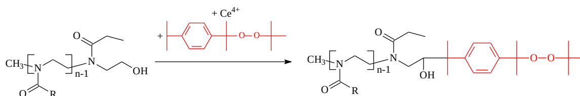
Рис.1. Схема отримання пероксидовмісного поліоксазоліну
