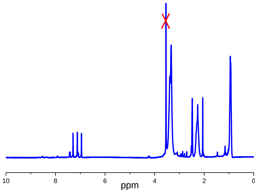
Рис.3. Спектр ЯМР полі(2-етилполіоксазоліну) з кінцевою пероксидною групою
