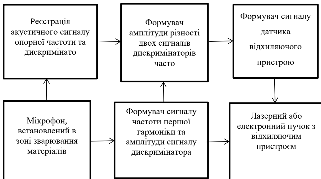
Рис. 1. Функціональна електрична схема датчика для автоматичного наведення на стик лазерного або електронного промінню.
