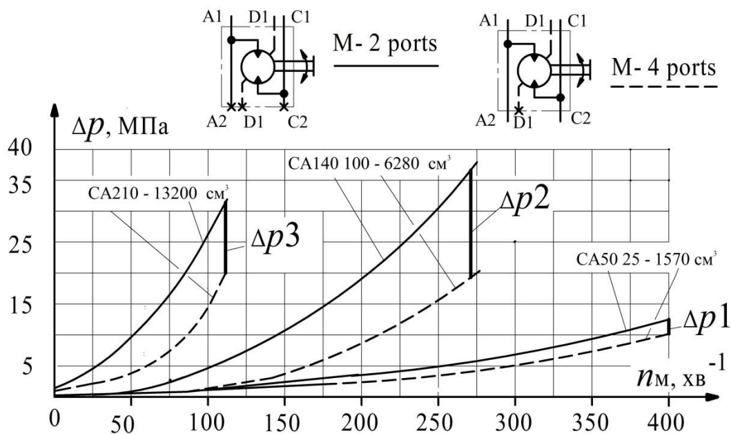
Рис. 3. Втрати (перепад тисків) холостого ходу гідромоторів Comract-CA залежно від кількості використовуваних отворів (2 або 4) для повідомлення з магістралями високого тиску (насоса) та зливу в гідробак
