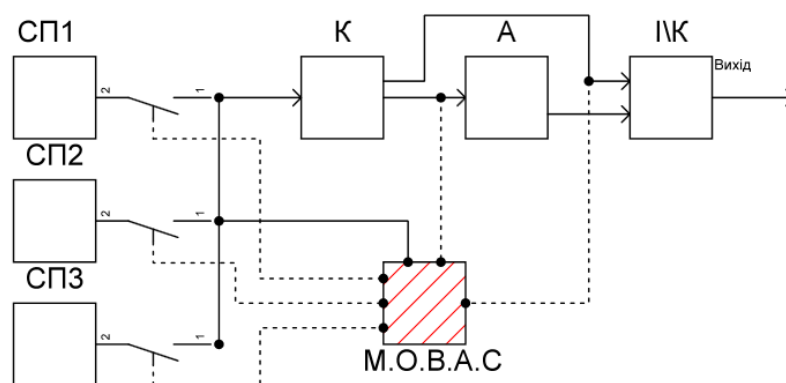
Рис. 3. Структурна схема автономної сонячної електростанції з регулюванням кількості СП в активному режимі. Де ІК – інвертор, інвертор-конвертор, М.О.В.А.С – система моніторингу, порівняння та відключення активних сонячних панелей.
