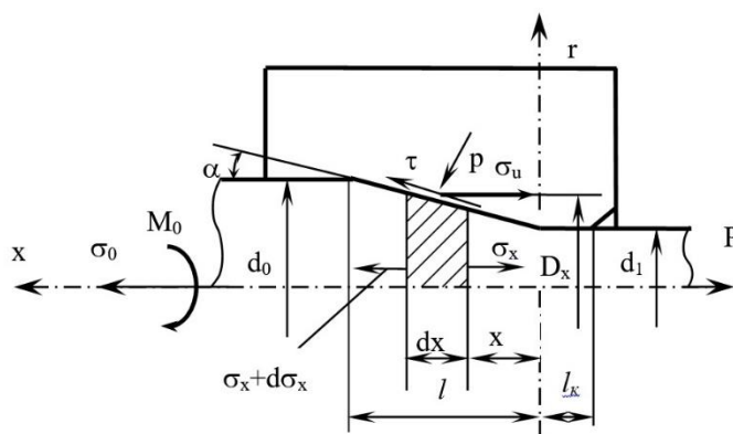
Рис. 1. Схема осередку деформації при волочінні профілю з віброколиваннями
