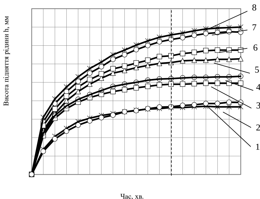
Рис. 1. Залежність висоти капілярного підняття рідини від часу у пробах текстильних матеріалів: 1 -арт. 521352; 2 - арт. 72040; 3 - арт. 52119; 4- арт. 44033; 5 - арт. 62082; 6 - арт. 63038; 7 - арт. 72471; 8 - арт. 63034.
