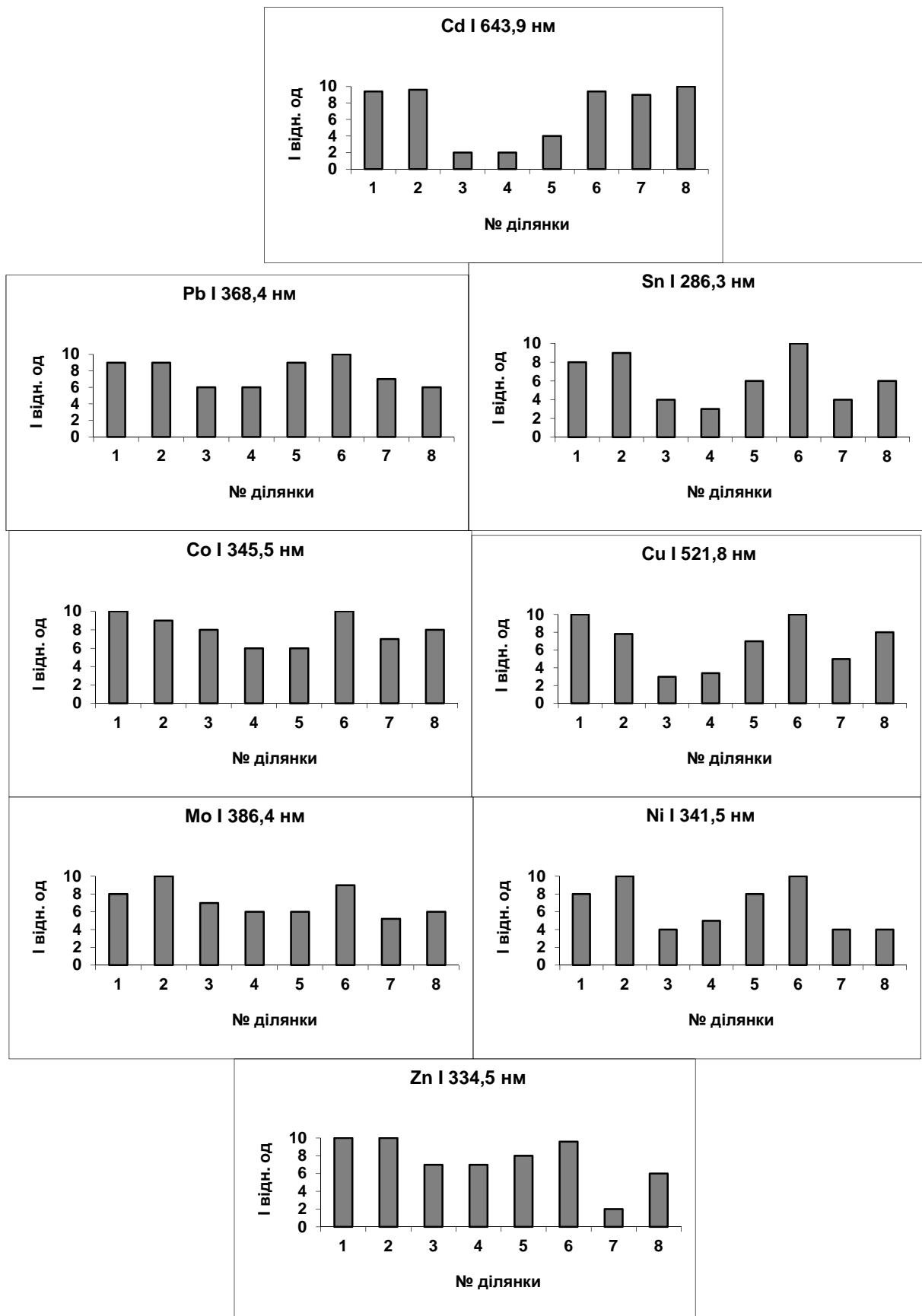
Рис.2. Діаграми валового вмісту ВМ на ділянках придорожньої смуги автодороги Чоп-Ужгород, отримані методом ІФС.
