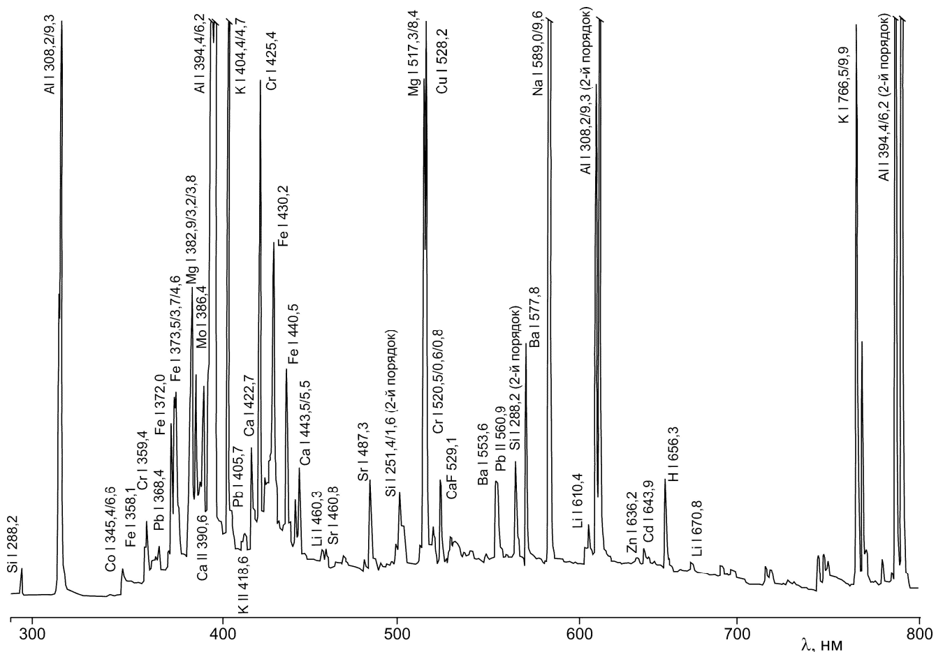
Рис.1. Спектрограма іон-фотонної емісії для ґрунту з ділянки №5.
