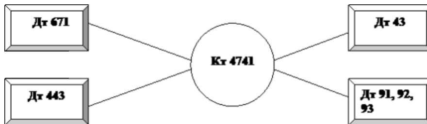
Рис. 4. Порядок відображення на рахунках бухгалтерського обліку формування інноваційного фонду
