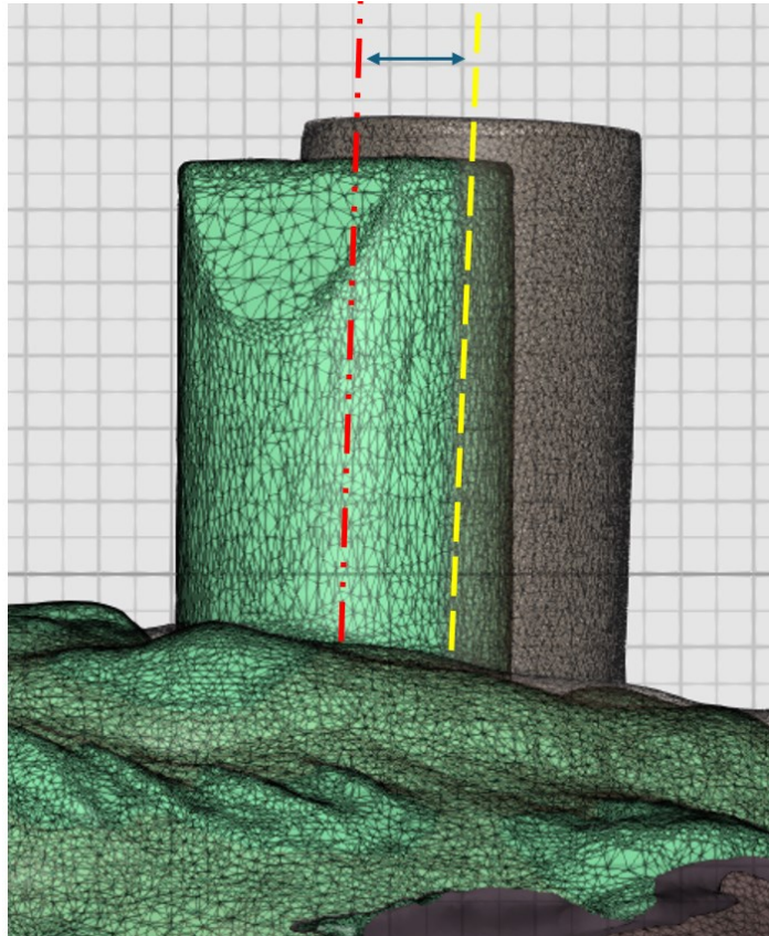
Рис. 2. Схематичне зображення центроїдних відхилень скан-абатментів на досліджуваному скані відносно референтної цифрової мастер-моделі (з клінічної практики та експериментальних досліджень Гончарук-Хомин М.Ю.)
