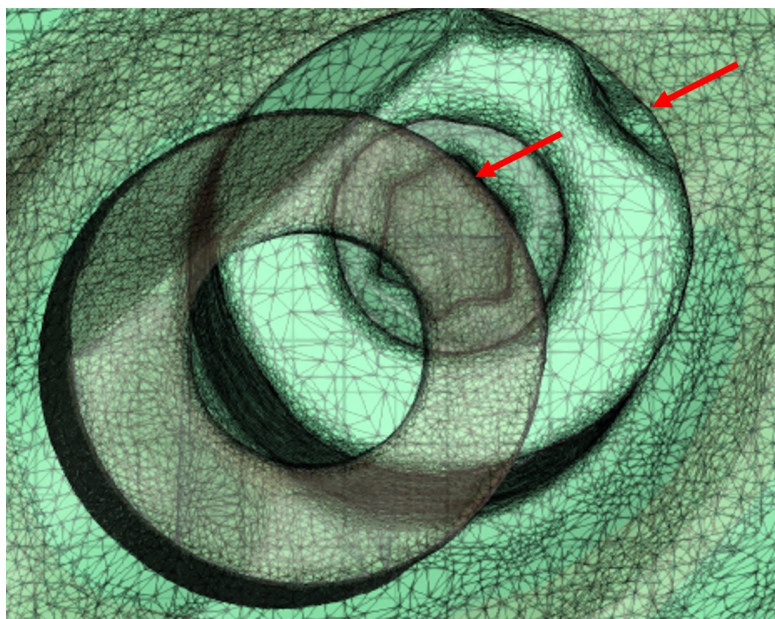
Рис. 3. Схематичне зображення відмінностей поверхонь скан-абатментів на досліджуваному скані відносно референтної цифрової мастер-моделі (з клінічної практики та експериментальних досліджень Гончарук-Хомин М.Ю.)
