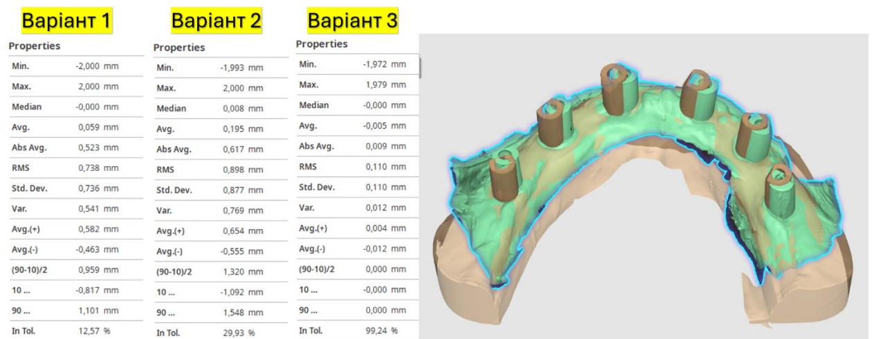
Рис. 8. Обрахунок сукупності статистичних параметрів (максимальних відхилень, значень медіани, середніх похибок, стандартних відхилень, варіації, середньоквадратичних похибок) для квантифікації точності реєстрації положення скан-абатментів за результатами суміщення досліджуваного скана та цифрової мастер-моделі
