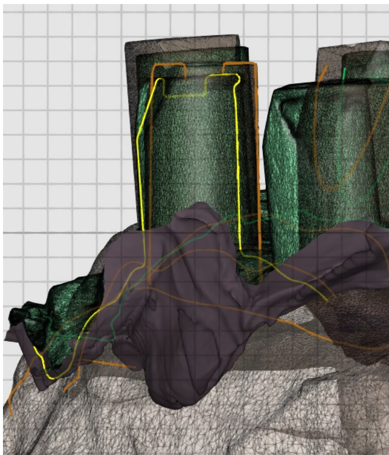
Рис. 7. Схематичне зображення відмінностей положення скан-абатментів на досліджуваному скані та цифровій мастер-моделі з реалізацією функції крос-секціонування та візуалізацією відмінностей площинних контурів
