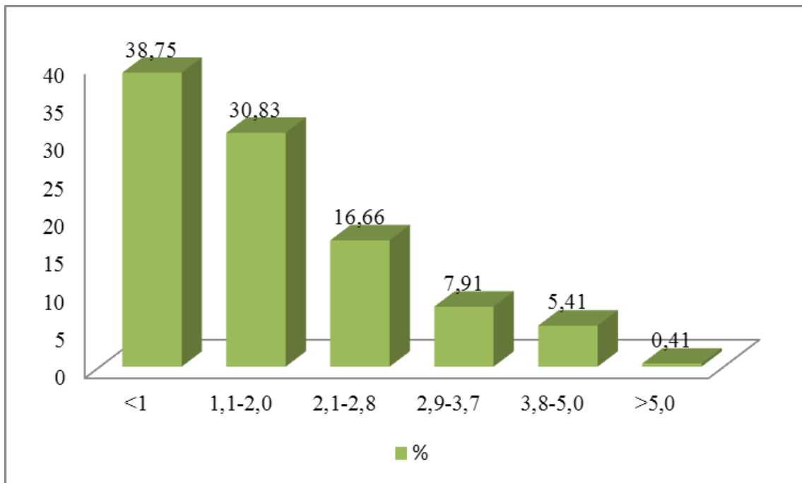
Рис. 4 – Горизонтальне розчленування масиву Оаш, км/км 2
