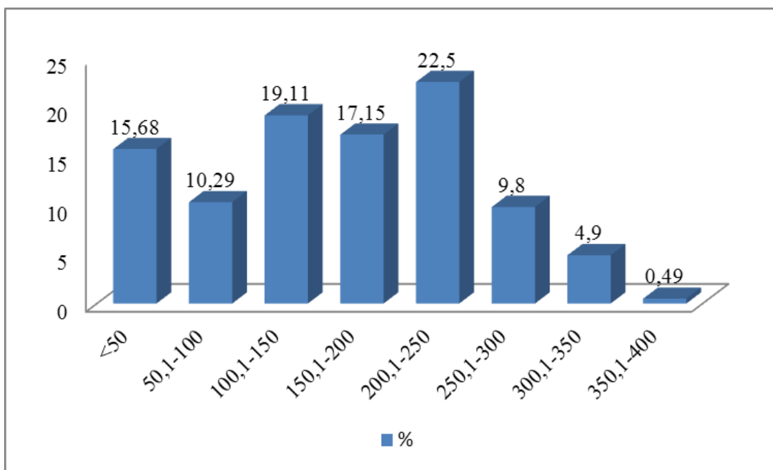
Рис. 3 – Вертикальне розчленування масиву Оаш, м/км 2
