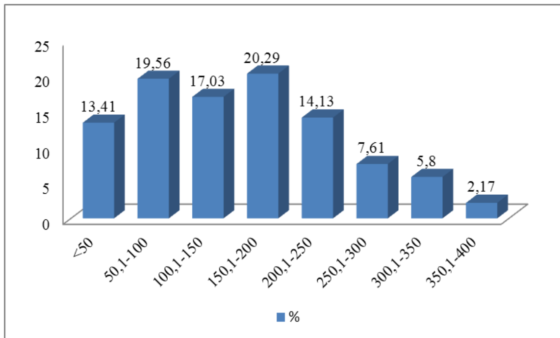
Рис. 1 – Вертикальне розчленування хребта Тупий, (м/км 2 )
