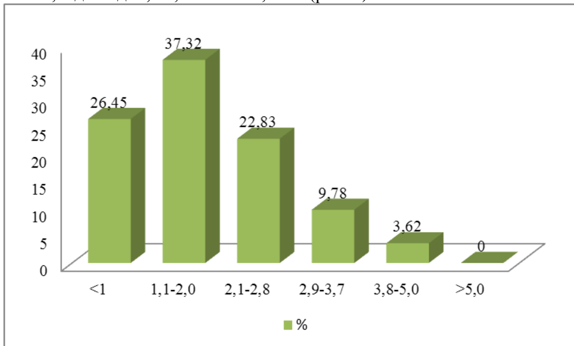
Рис. 2 – Горизонтальне розчленування хребта Тупий, км/км 2
